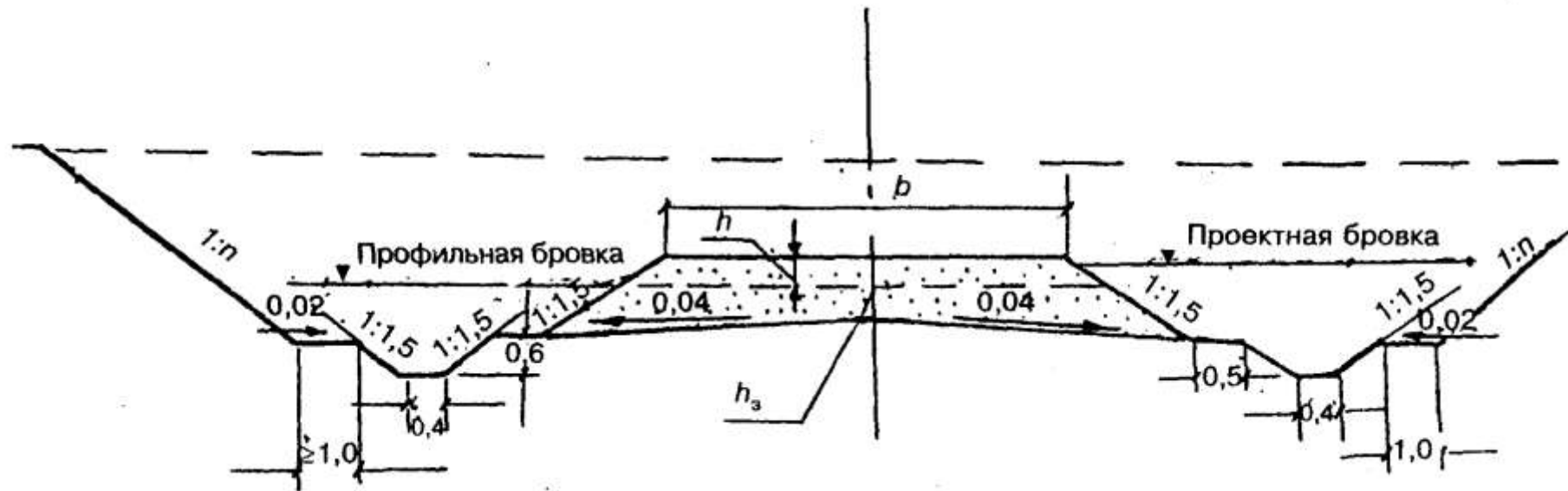
Рисунок 10.5 — Поперечный профиль выемки глубиной до 12 м в мелких и пылеватых песках, в глинистых грунтах с W_L \leq 0,23 и в легковыветривающихся скальных
