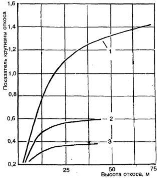
Рисунок P.2 — Зависимость оптимальной крутизны откосов выемок от их высоты для сухих косогоров
