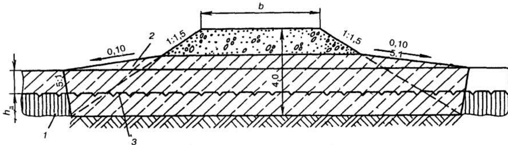
Рисунок 20.6—Схема устройства насыпи над подземным льдом, залегающим на глубине, равной мощности деятельного слоя
