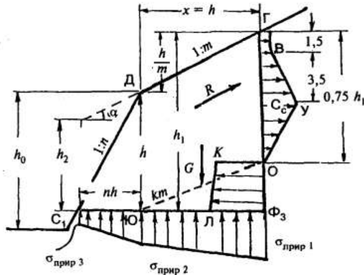
Рисунок P.3 — Расчетная схема для определения устойчивости откоса выемки в мокром лессовом косогоре
