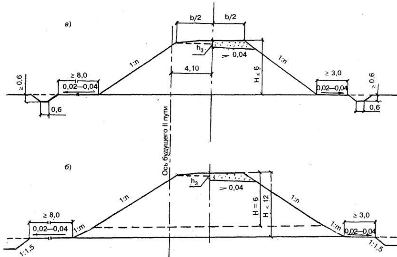
а — насыпь без защитного слоя H \leq 6 м; б — то же, высотой от 6 до 12 м; в — насыпь с защитным слоем H \leq 6 м; г — то же, высотой от 6 до 12 м Рисунок 7.1 — Поперечные профили насыпей из недреняющих грунтов при поперечном уклоне местности не круче 1:5
