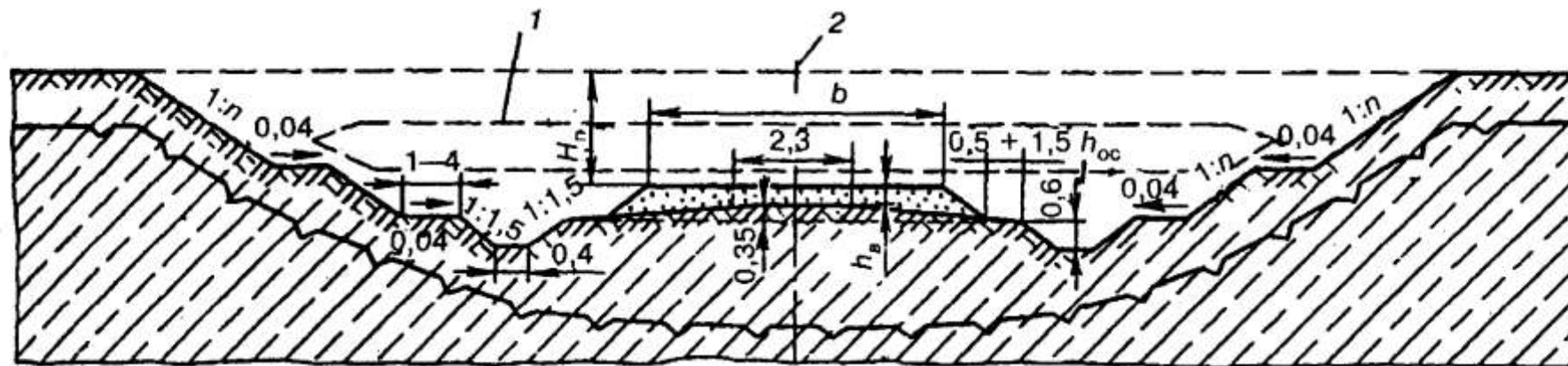
Рисунок 20.6—Схема устройства насыпи над подземным льдом, залегающим на глубине, равной мощности деятельного слоя
