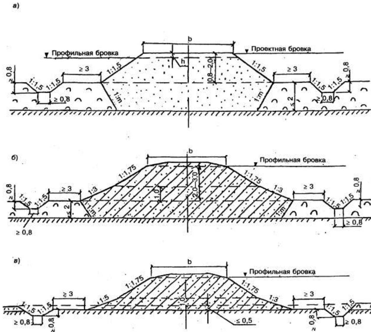
Рисунок 8.1 — Поперечные профили насыпей высотой до 3 м с предварительным выторфовыванием на болотах 1 типа глубиной до 2 м при поперечном уклоне основания не круче 1:10
