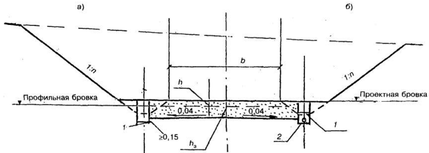
а — с железобетонным лотком; б — с лотком и дренажем мелкого заложения; h_3 — толщина слоя замены глинистого грунта дренирующим; 1 — водоотводный лоток; 2 — дренаж мелкого заложения
