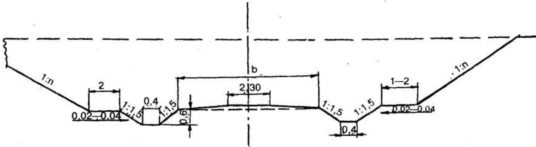
Рисунок 10.5 — Поперечный профиль выемки глубиной до 12 м в мелких и пылеватых песках, в глинистых грунтах с W_L \leq 0,23 и в легковыветривающихся скальных
