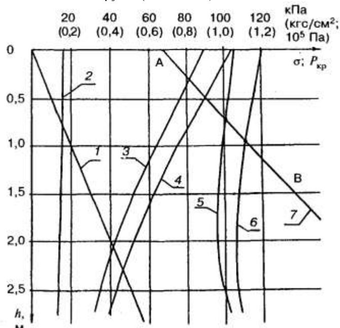
Напряжения от: 1 — собственного веса грунта; 2 — верхнего строения пути; 3, 4 — поездной нагрузки для 4- и 8-осных вагонов при скоростях движения 120 км/ч ( P_{oc} = 30 тс/ось); 5, 6 — суммарные напряжения при 4- и 8-осных вагонах; 7 — прямая изменения несущей способности грунта P_{кр}
