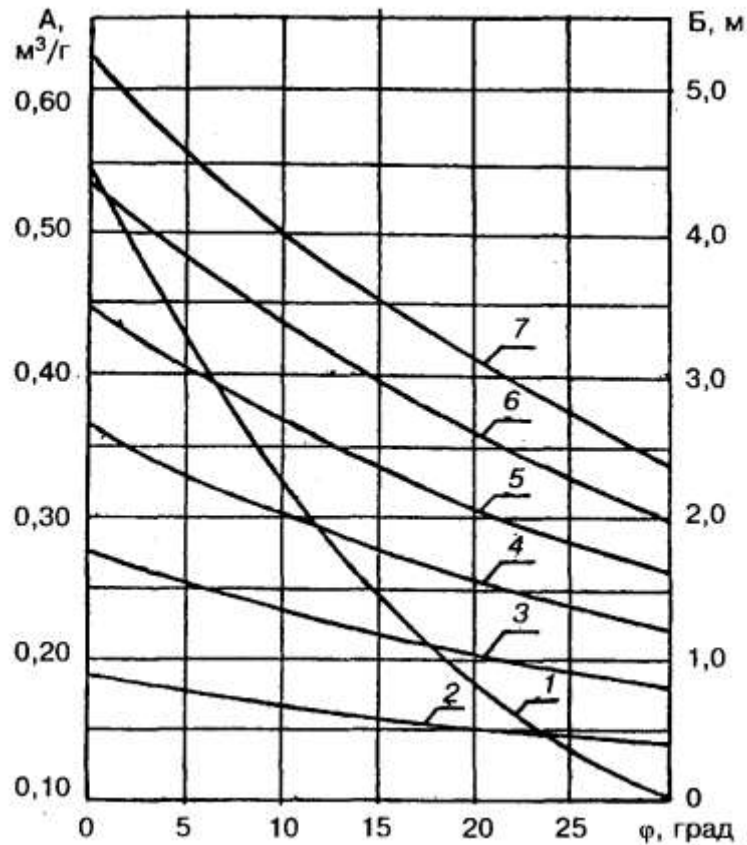
1 — кривая зависимости А от \phi ; 2—7 — кривые зависимости параметра В от \phi при С, равном соответственно 0,5; 1,0; 1,5; 2,0; 2,5; 3,0 тс/м 2
