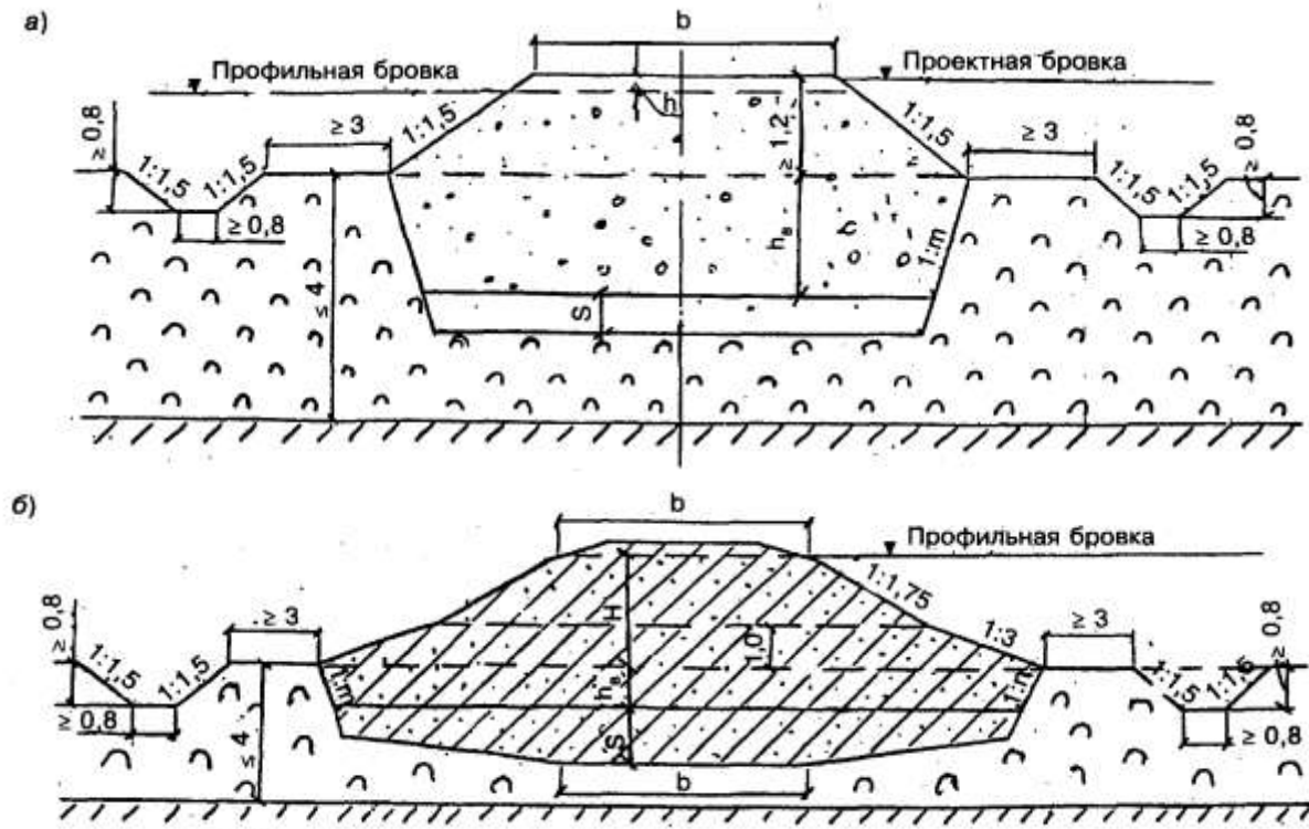
а — из дренирующих грунтов; б—из мелких и пылеватых песков, песчанистых супесей; 1 : m — крутизна откосов траншеи выторфовывания (от 1:0 до 1:0,5 ); h_г — глубина траншеи выторфовывания; S — осадка насыпи Рисунок 8.2 — Поперечные профили насыпей высотой от 2 до 3 м с частичным выторфовыванием на болотах I типа глубиной от 2 до 4 м при поперечном уклоне минерального дна болота не круче 1:10
