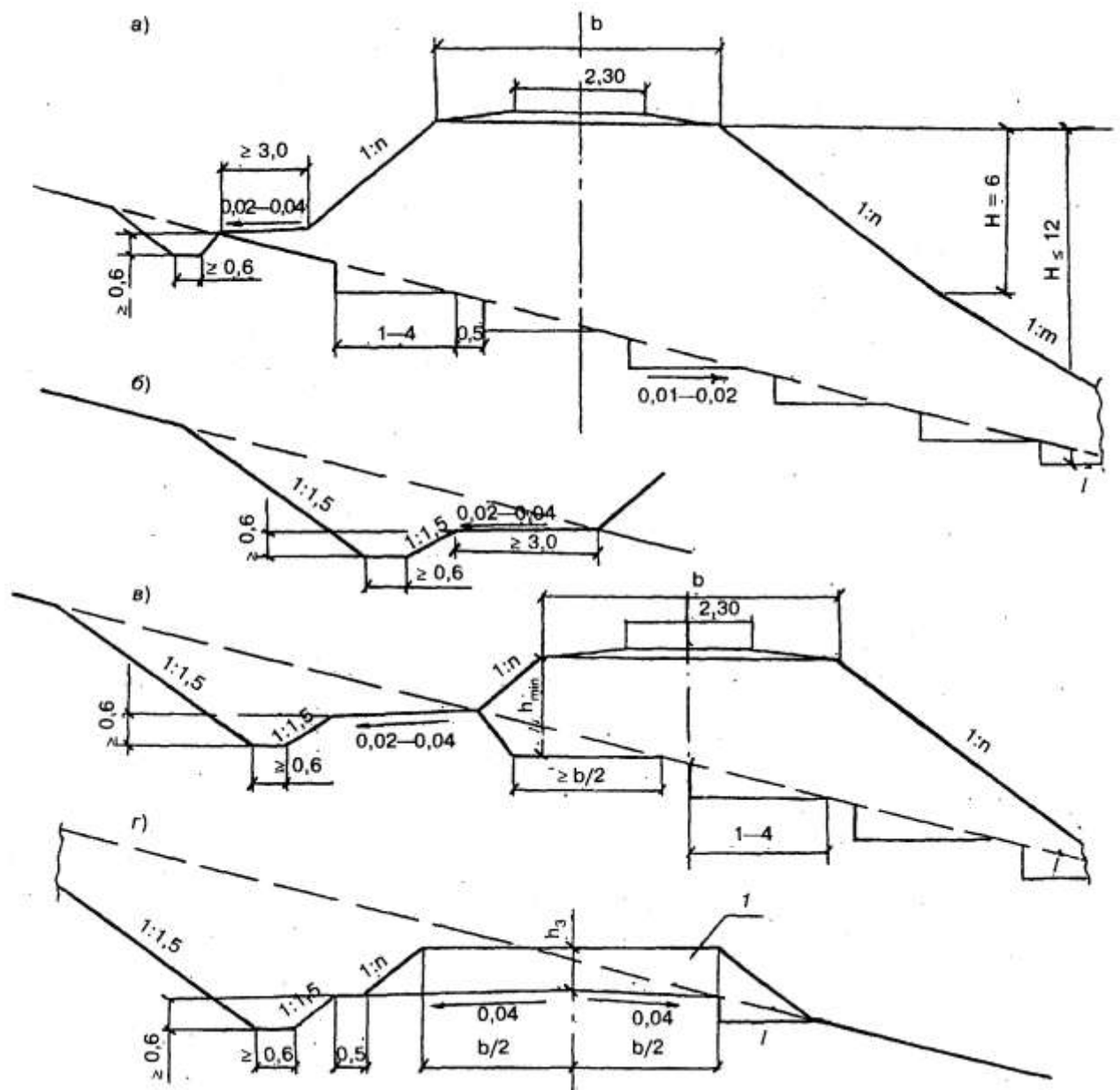
а — насыпь высотой низового откоса до 12 м; б — деталь нагорной канавы с бермой в грунте естественного сложения; в — низкая насыпь на косогоре; г — полунасыпь-полувыемка; l — ширина нижнего уступа определяется из условия возможности уплотнения грунтов нижней части насыпи; 1 — защитный слой
