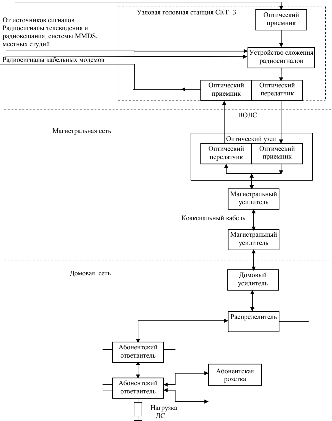
Рисунок 4.3 - Структурная схема городской кабельной распределительной сети СКТ-3
