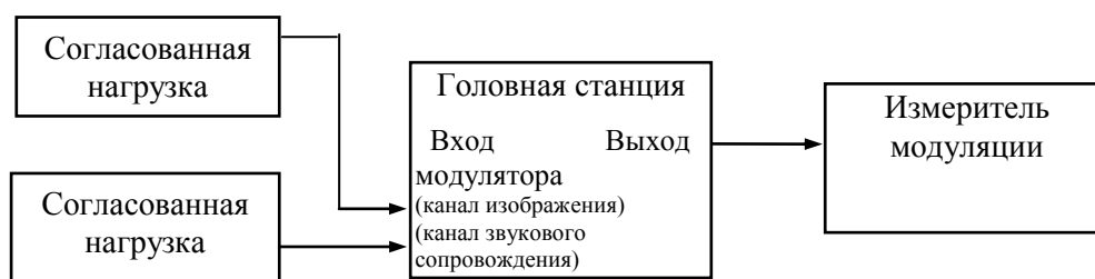
Рисунок 7.24 Структурная схема для определения отношения сигнала к фоновой помехе
