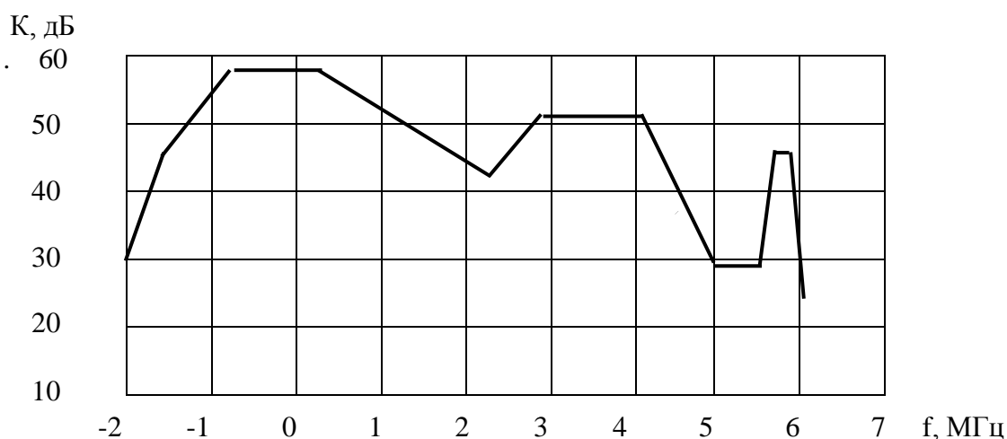
Рисунок 5.1 - Кривая защитных отношений для системы вещательного телевидения
