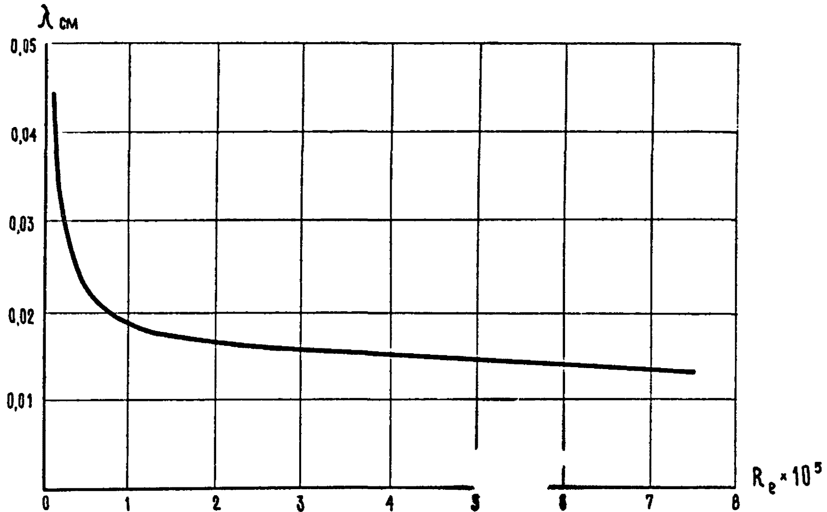
Рис. 3.2. ЗАВИСИМОСТЬ КОЭФФИЦИЕНТА ГИДРАВЛИЧЕСКИХ СОПРОТИВЛЕНИЙ ОТ ЧИСЛА РЕЙНОЛЬДСА.
