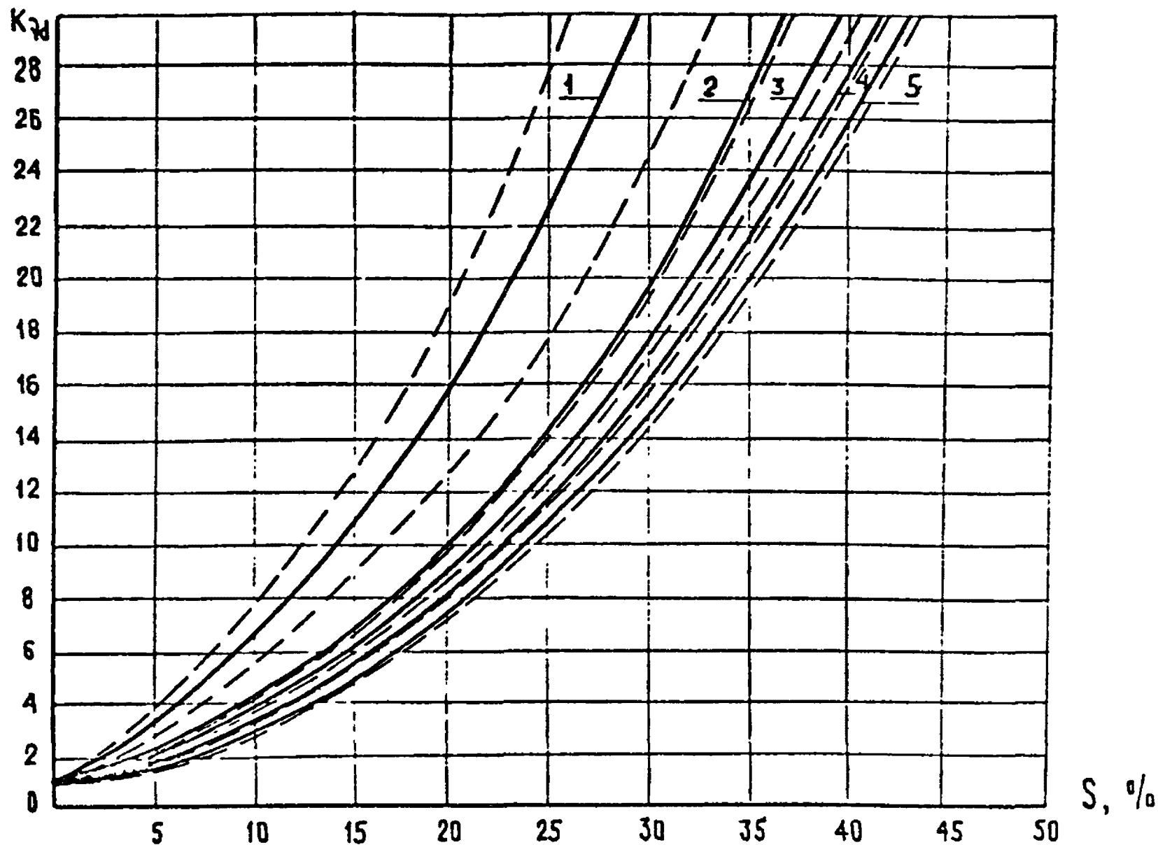
Рис. 3.3. ЗАВИСИМОСТЬ КОЭФФИЦИЕНТА K_{\Sigma} ОТ КОНЦЕНТРАЦИИ ПУЛЬПЫ И СРЕДНЕВЗВЕШЕННОЙ КРУПНОСТИ ТРАНСПОРТИРУЕМОГО МАТЕРИАЛА.
