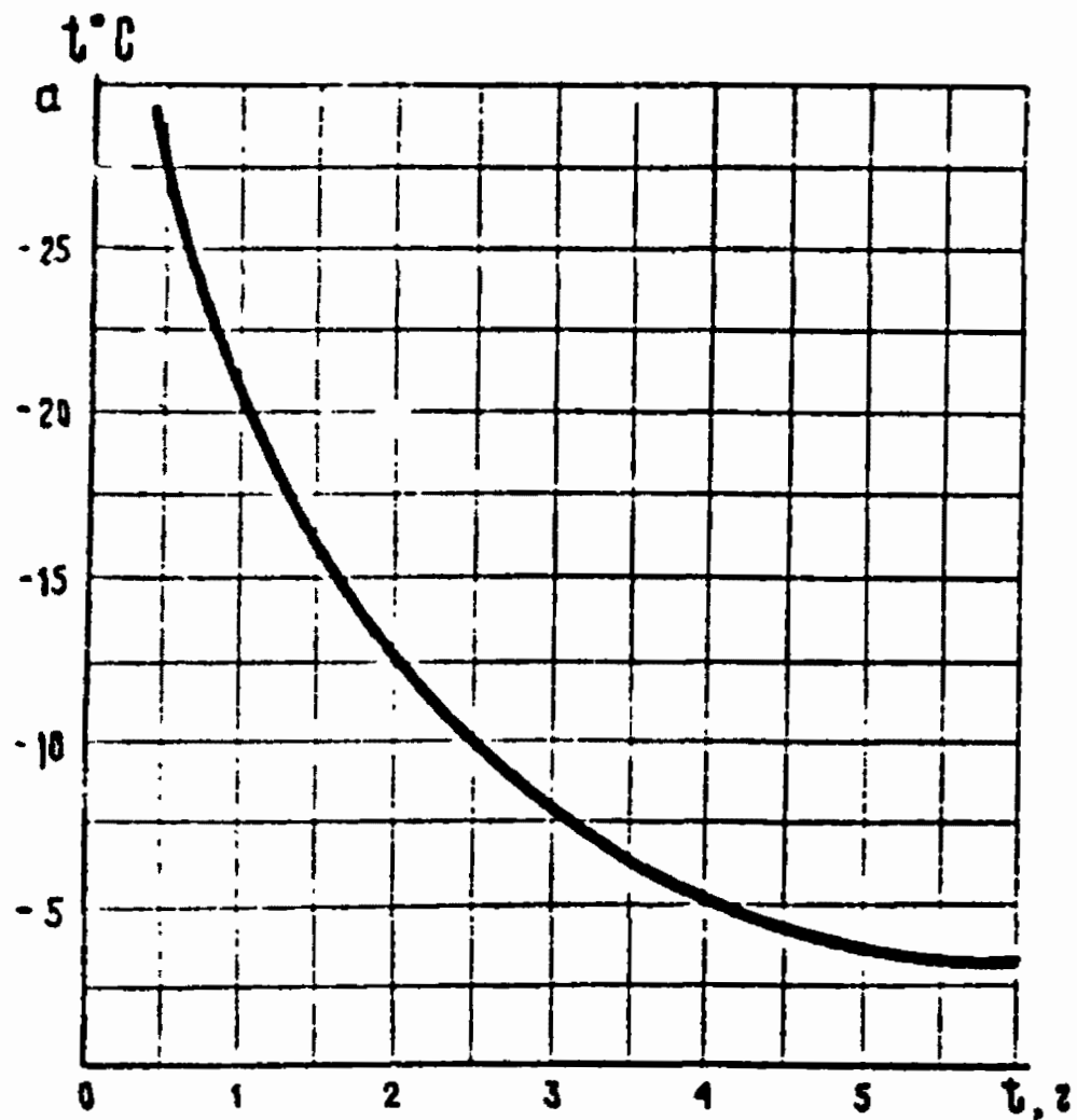
Рис. 6.1. ДОПУСТИМОЕ ВРЕМЯ НАХОЖДЕНИЯ ВОДЫ ИЛИ ПУЛЬПЫ В ТРУБОВОДЕ ДИАМЕТРОМ 300–600 мм В ЗАВИСИМОСТИ ОТ ТЕМПЕРАТУРЫ ОКРУЖАЮЩЕГО ВОЗДУХА ПРИ ОСТАНОВКЕ ГИДРОТРАНСПОРТА ( по данным ВОДГЕО , Госстрой СССР).
