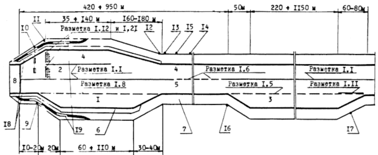
Рис.7.5. Элементы обустройства и принципиальная схема организации движения в зоне накопительных, посадочных и дополнительных полос для обгона:
