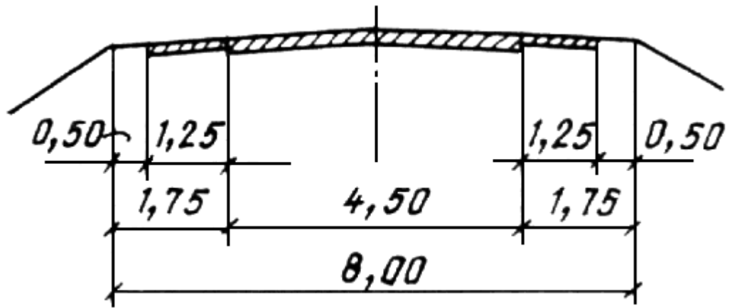
Рис. 2.5. Поперечный профиль автомобильной дороги II-с-а категории
