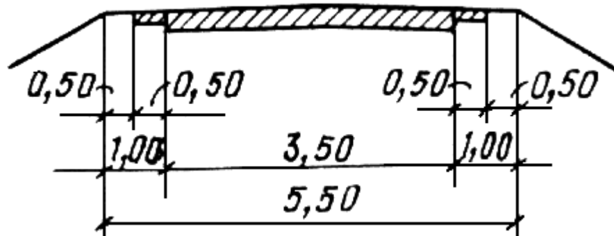
Рис. 2.6. Поперечный профиль автомобильной дороги II-с-б категории
