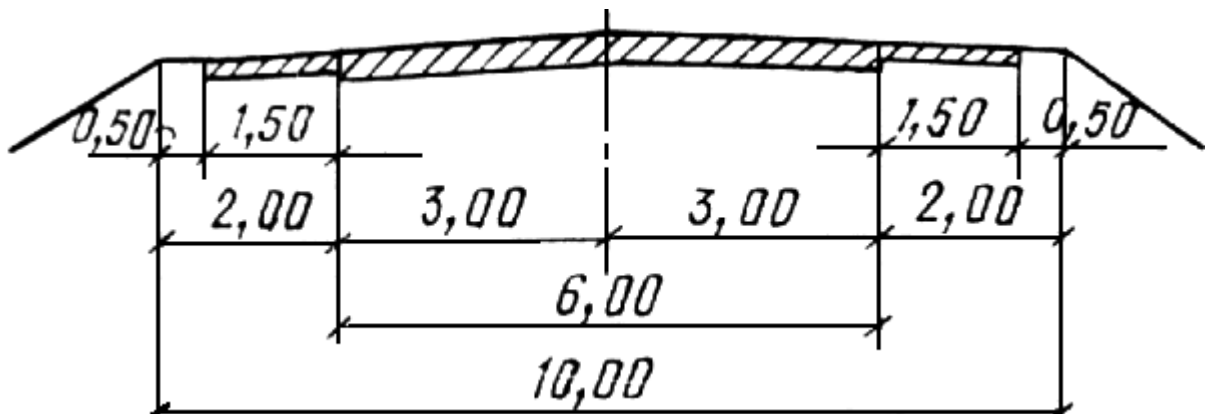
Рис. 2.3. Поперечный профиль автомобильной дороги IV-б и I-б категории
