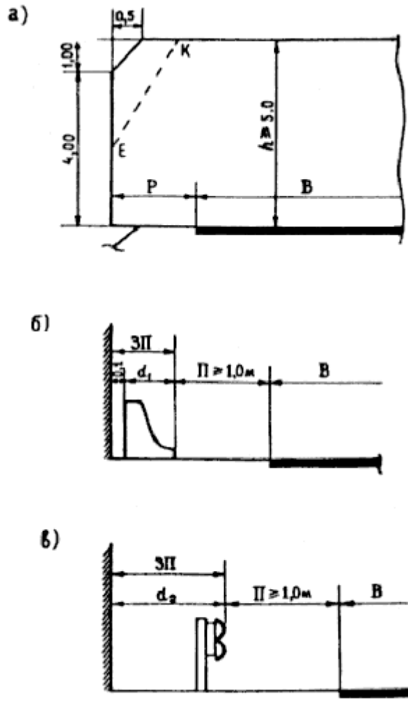
Рис. 6.2. Схемы габаритов приближения конструкций под путепроводами при проектировании новых автомобильных дорог (а), при реконструкции существующих автомобильных дорог с применением парапетных ограждений (б) и барьерных ограждений (в):
