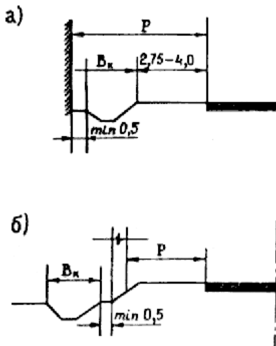
Рис. 6.3. Схема расположения боковых водоотводных канав (кюветов) в одном (а) и соседнем (б) пролетах с проезжей частью дороги
