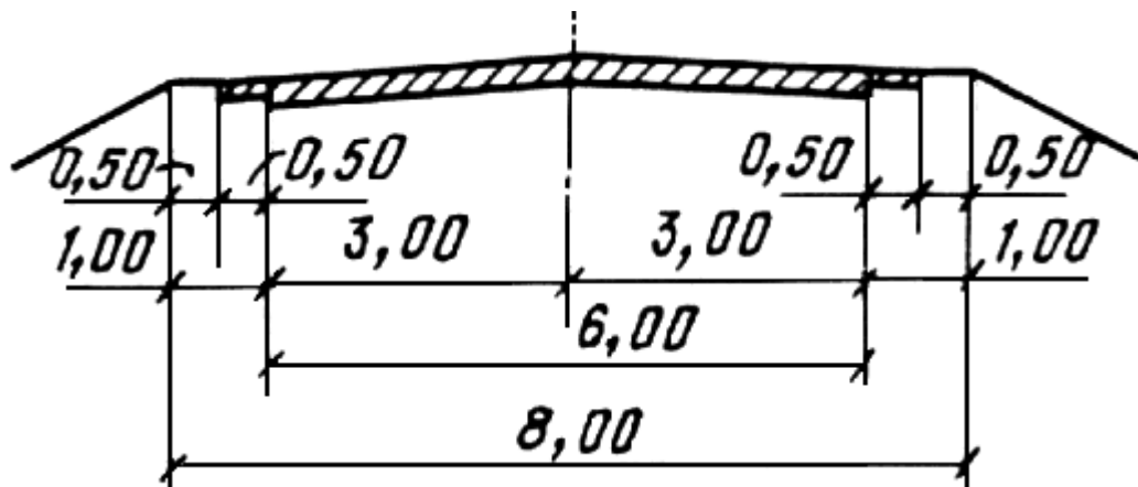
Рис. 2.4. Поперечный профиль автомобильной дороги IV-в и I-в категории
