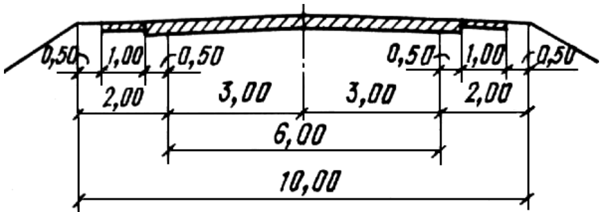
Рис. 2.2. Поперечный профиль автомобильной дороги IV-а и I-а категории
