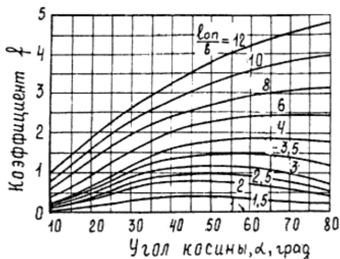
Рис.1. График для определения параметра f в формуле коэффициента косины
