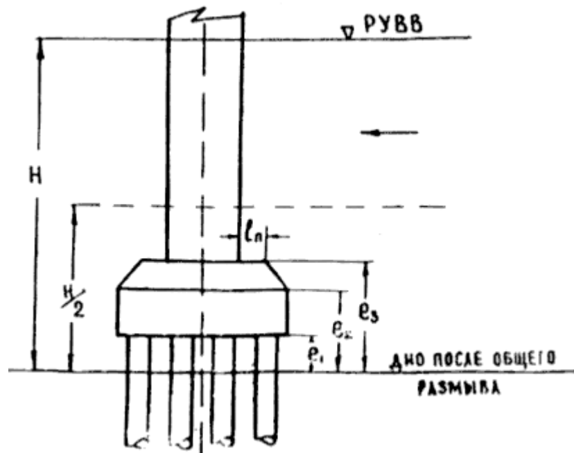
Рис.3. К расчету опор с переменным поперечным сечением
