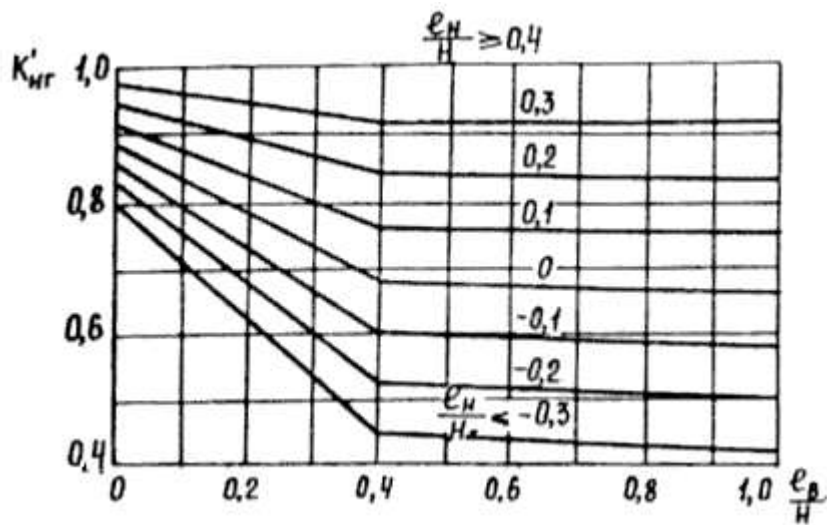
Рис.4. График для определения коэффициента K_{\text{ср}}
