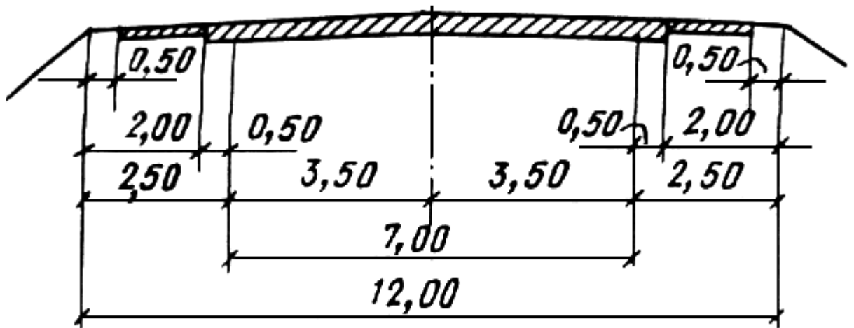
Рис. 2.1. Поперечный профиль автомобильной дороги III категории
