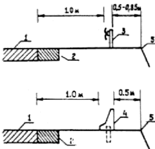
Рис. 7.2. Схема размещения ограждений на обочинах дорог:
