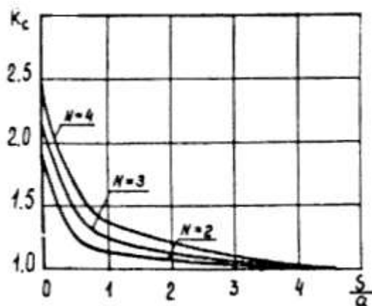
Рис. 5. График для определения коэффициента K_c
