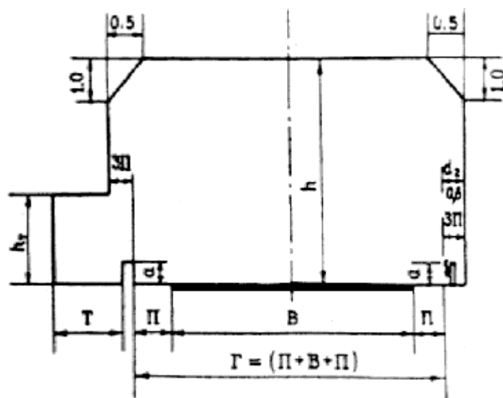
Рис. 6.1. Схема габаритов приближения конструкций на мостовых сооружениях:
