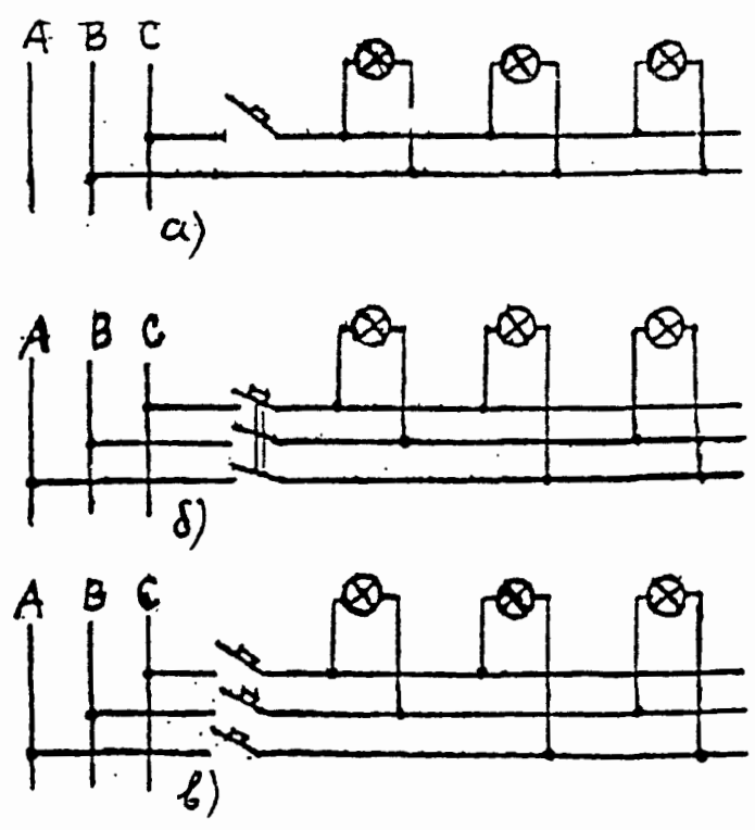
Рис.3. Схемы групповых линий при системах 3x220 и 220/127 В при питании ОП напряжением 220 В и отсутствии необходимости заземления или зануления ОП. а - двухпроводная двухфазная; б - трехпроводная трехфазная с трехполюсным автоматом; в - трехпроводная трехфазная с тремя однополюсными автоматами.
