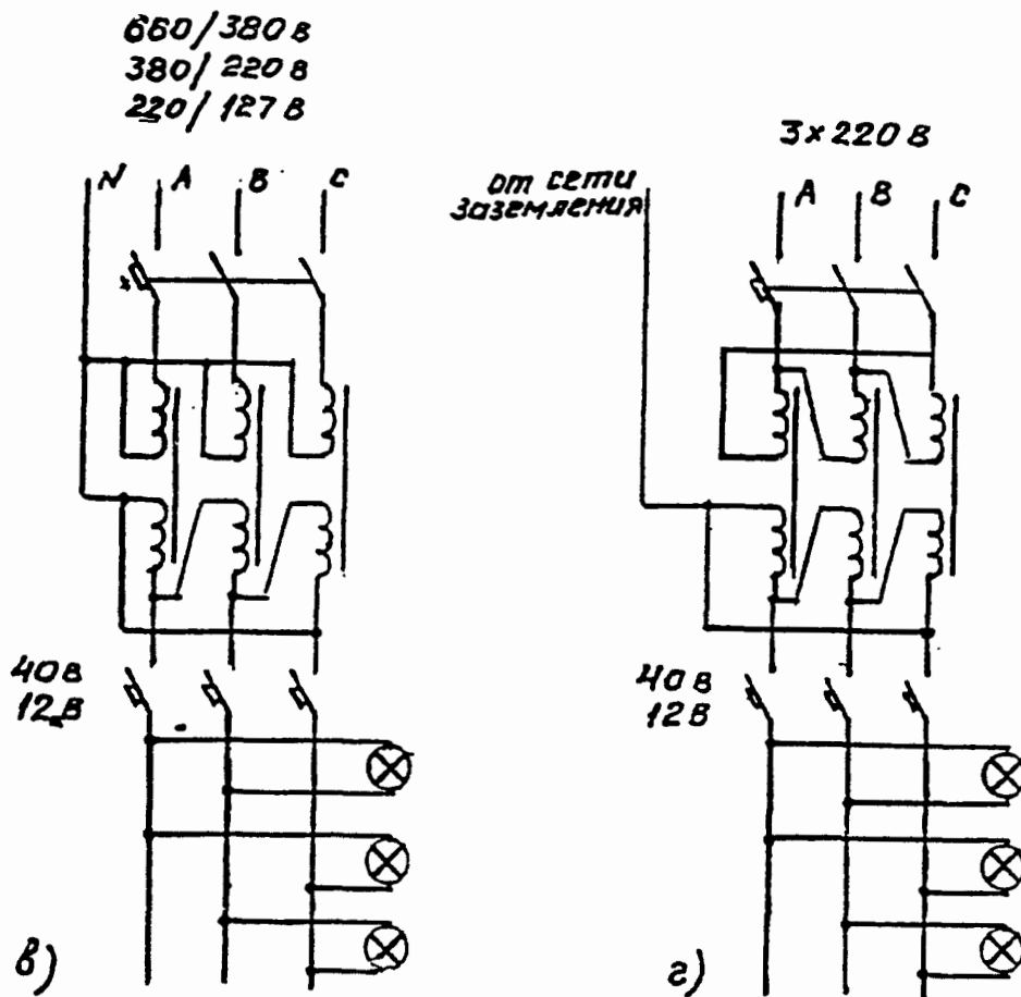
Рис. 4. Схемы сети малого напряжения при питании от трансформаторов: а, б - однофазных; в, г - трехфазных.
