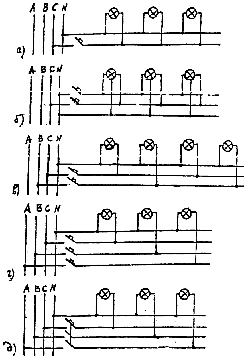
Рис. 1. Схемы групповых линий при системах напряжения напряжения 660/380, 380/220 и 220/127 В и питания ОП напряжением соответственно 380, 220 и 127 В.
