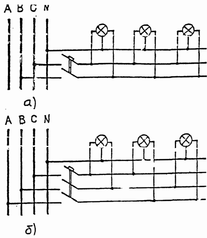
Рис.2. Схемы групповых линий при системе 380/220 и 220/127 В и питания ОП напряжением 380 и 220 В. а - трехпроводная двухфазная; б - четырехпроводная трехфазная.
