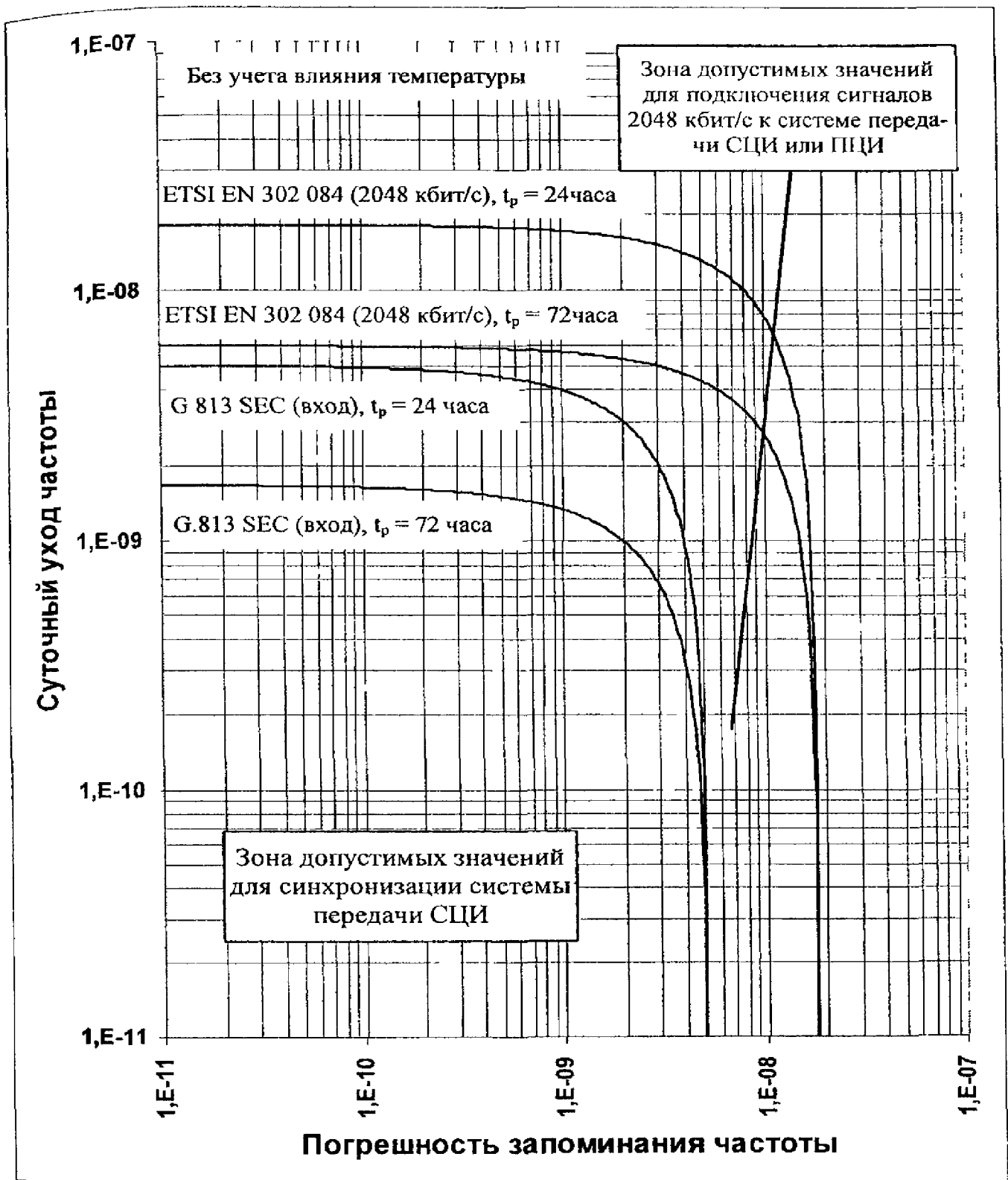
Рисунок 5.1 - Соотношения между относительной погрешностью запоминания и относительным уходом частоты за сутки для генератора в режиме удержания по критерию МОВИ
