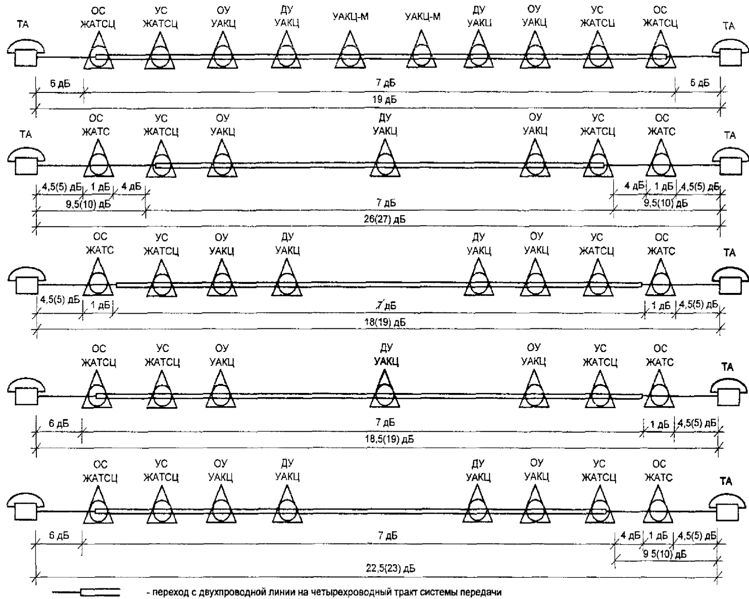
Рис. 3.7. Распределение норм затухания на междугородней сети ОБТС
