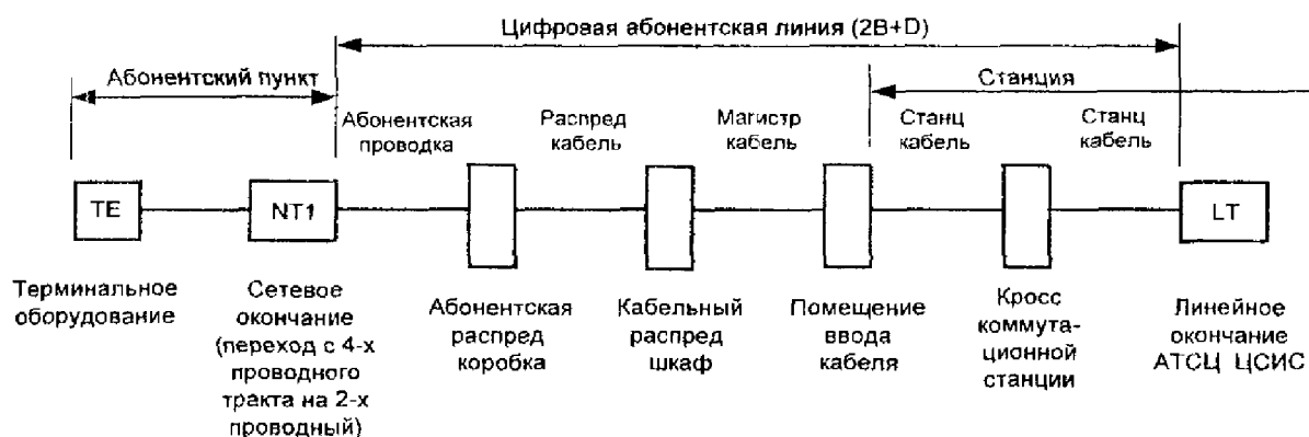
Рисунок 3.1 Структура цифровой абонентской линии (2В+D) ЦСИС
