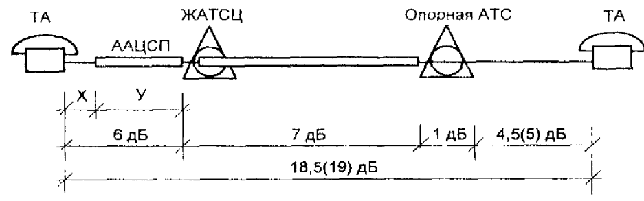
Рис. 3.5 Распределение норм затухания при включении ЖАТСЦ в местную сеть ТфОП по соединительным линиям (каналам)
