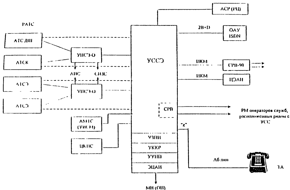
Рисунок 6.4 - Структурная схема организации связи со спецслужбами с использованием оборудования УИСЭ-0 и УССЭ
