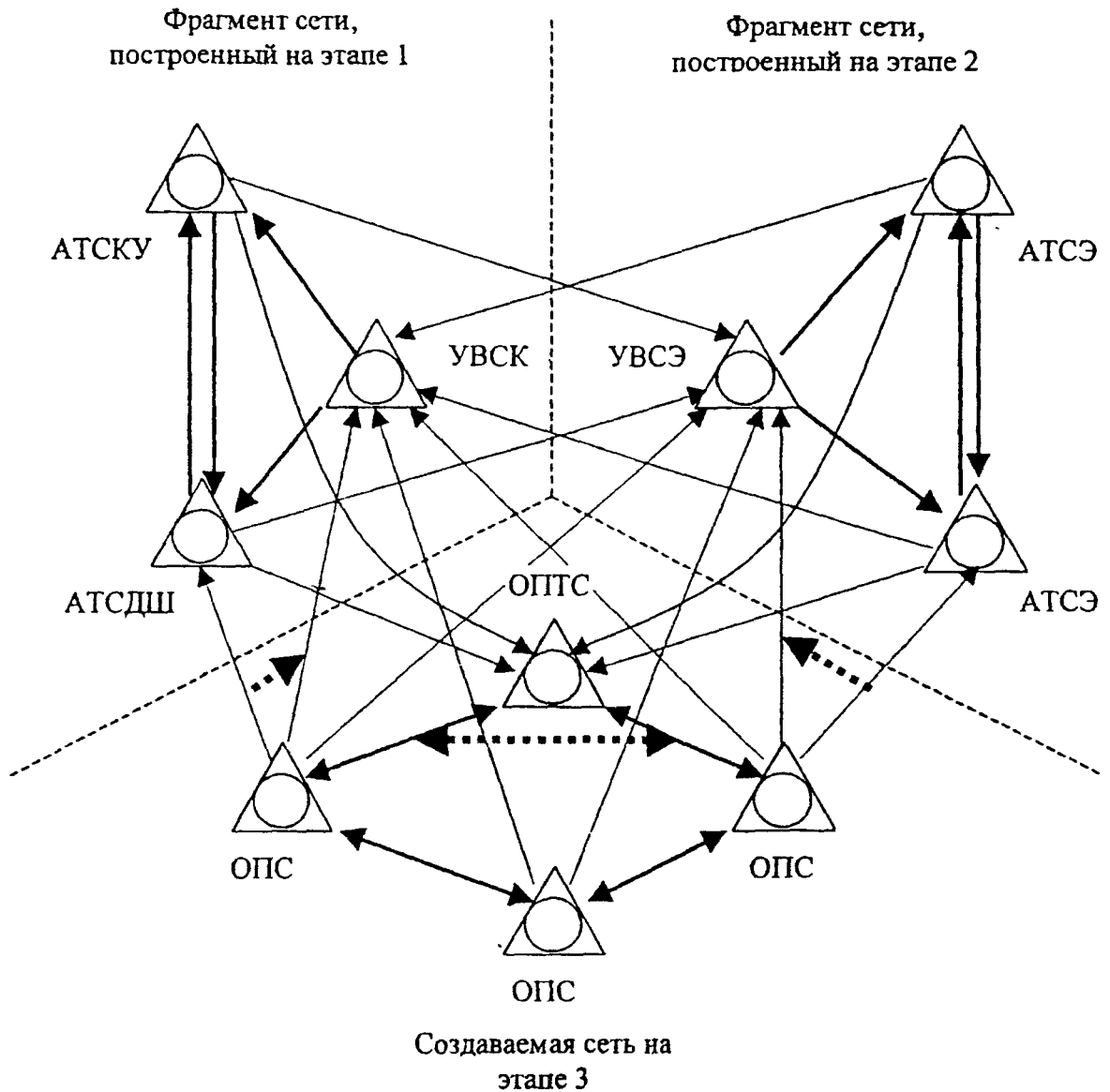
Рисунок 6.1 - Построение ГТС на переходном этапе, где:
