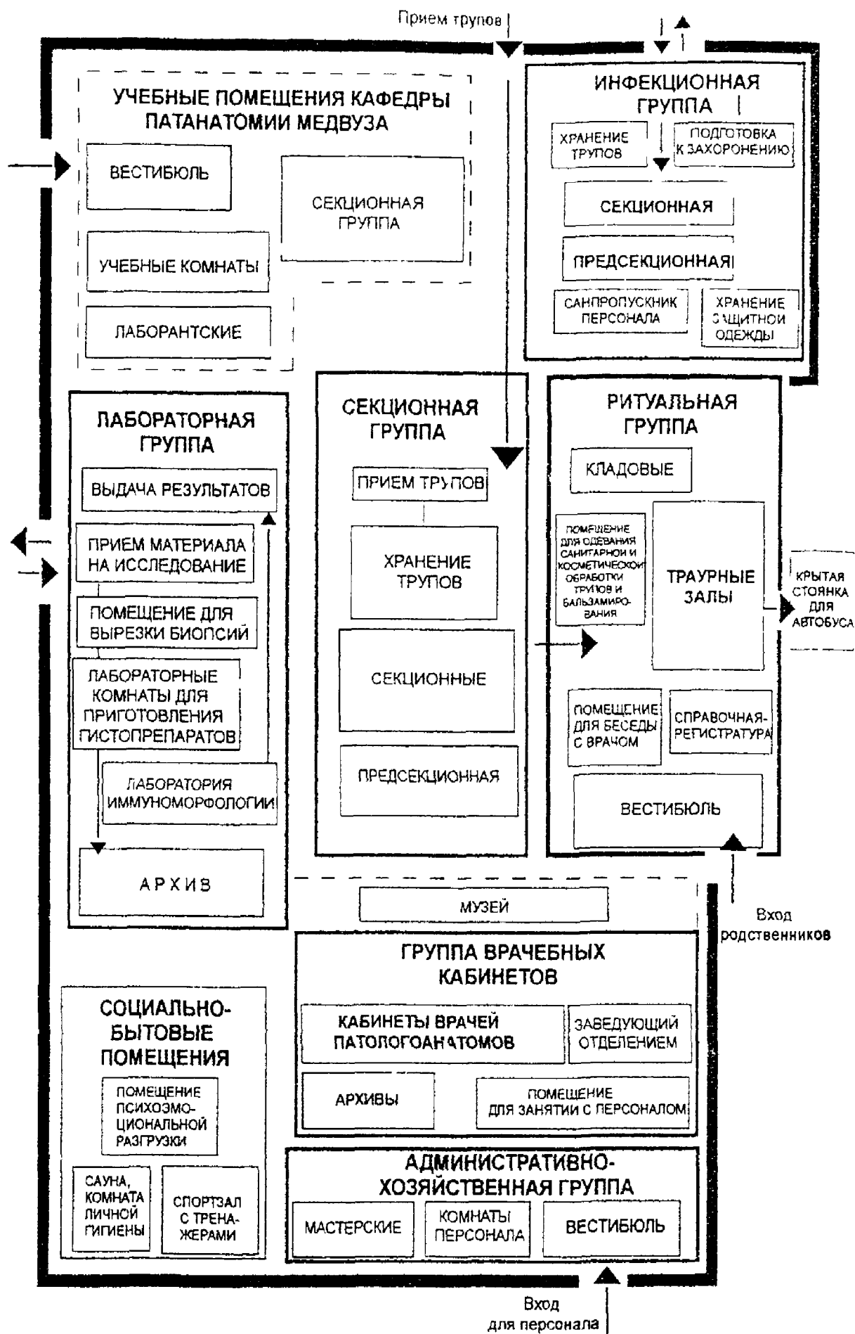
Рис 2.1 Схема взаимосвязей основных помещений патологоанатомического отделения
