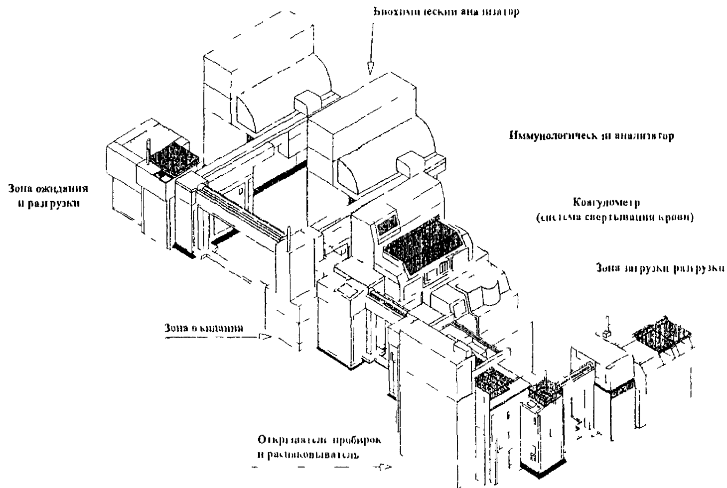
Рис 1.2 Вариант компоновки оборудования лаборантской для биохимических гормональных иммунологических исследований и для коагулологии Габариты оборудования - 3,5 x 8,0 м
