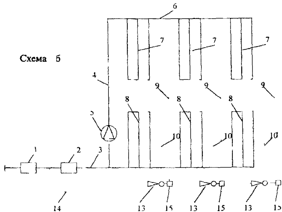
Рис 4 1 Принципиальная схема двухзонной системы горячего водоснабжения с элеваторным побуждением циркуляции в нижней зоне
