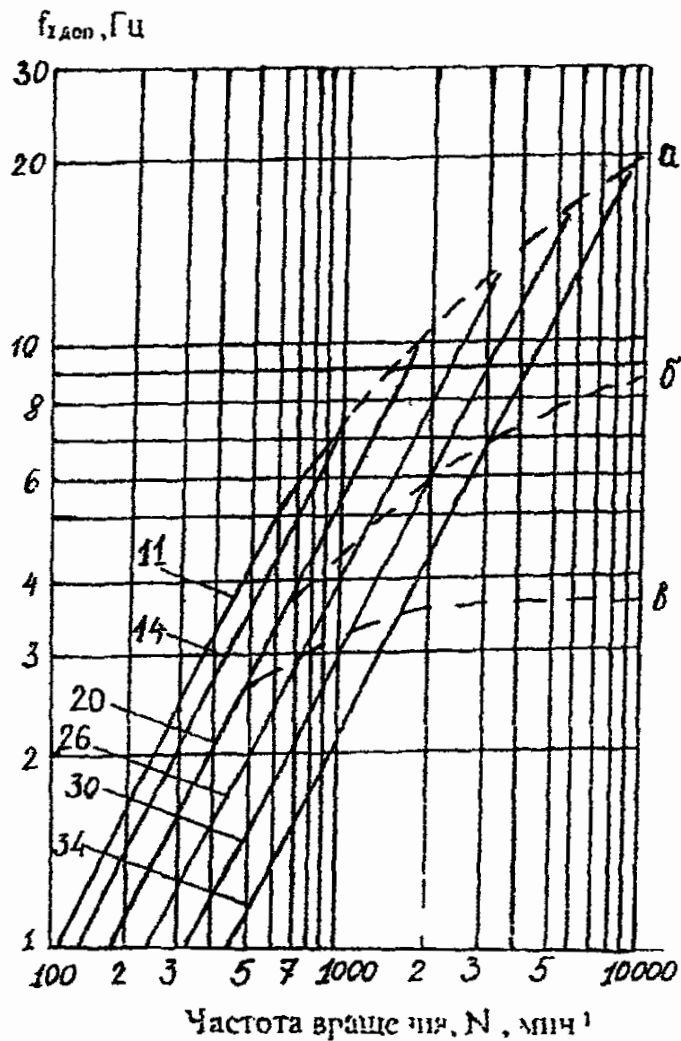
Рис. 1 Допустимая частота собственных вертикальных колебаний виброизолированного агрегата а - подвальные этажи; б - тяжёлые железобетонные перекрытия ( G \geq 500 \text{ кг/м}^2 ); в - лёгкие бетонные перекрытия ( 500 > G > 200 \text{ кг/м}^2 ); (цифры внутри графика указывают требуемую эффективность виброизоляции \Delta L_{тр} , дБ).
