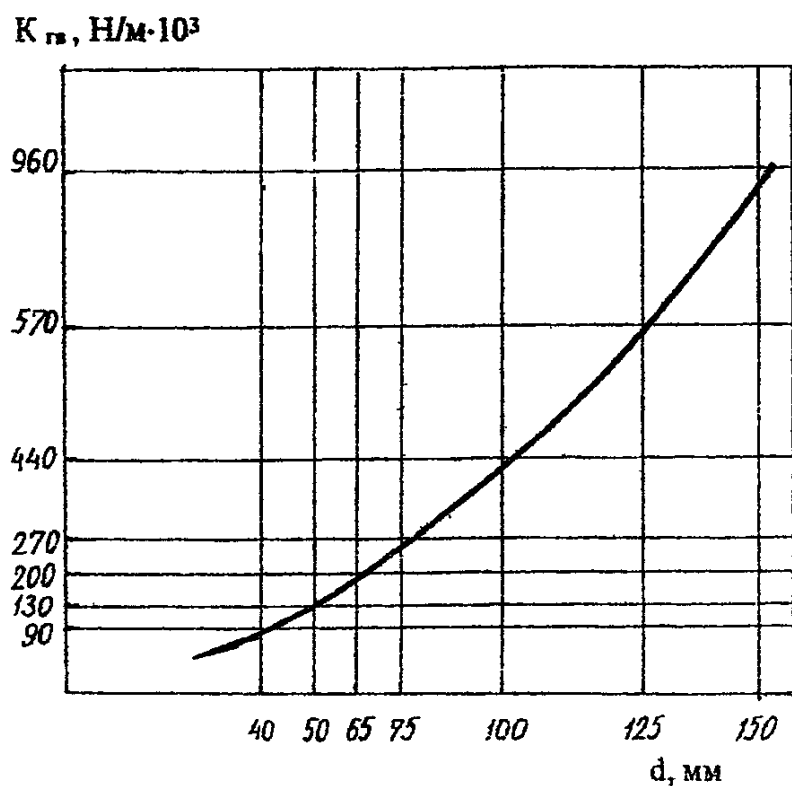
Рис. 4. Зависимость продольной динамической жёсткости K_{гв} гибких вставок ВГН от их внутреннего диаметра ( по данным СантехНИИпроекта)
