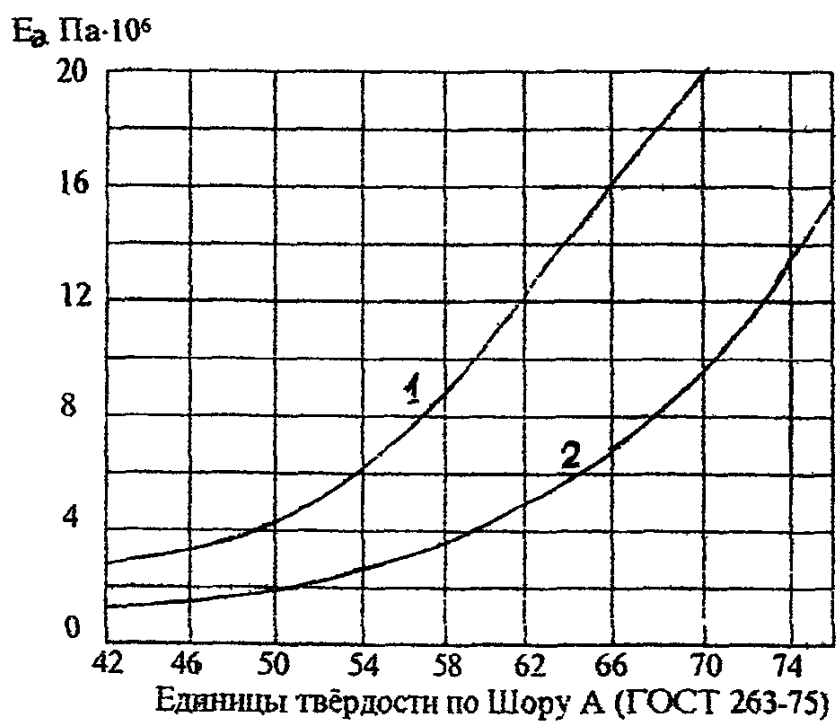
Рис.3. Зависимость динамического модуля упругости резины от твёрдости.
