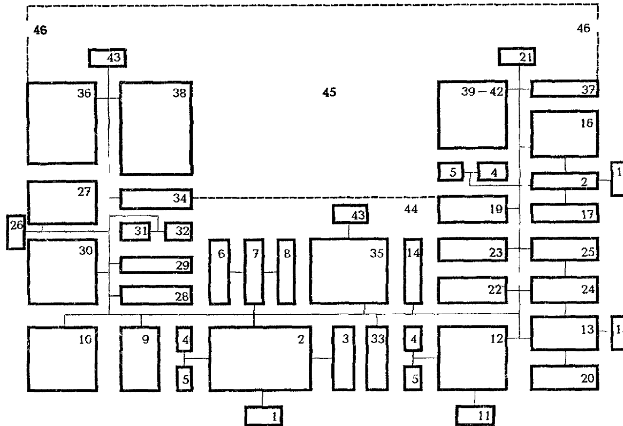
Административно-бытовое и обрядовое здание кладбища. Функционально-технологическая схема.
