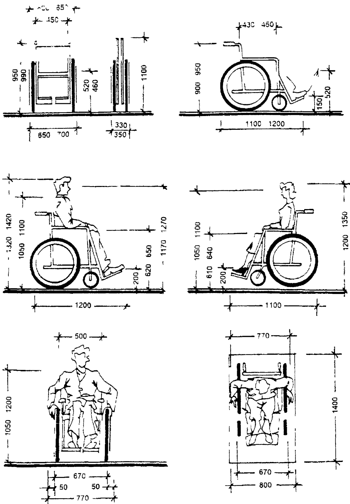
РИС 3 6 ГАБАРИТЫ КОЛЯСОК ПРИМЕНЯЕМЫХ ДЛЯ ПЕРЕДВИЖЕНИЯ ШКОЛЬНИКОВ
