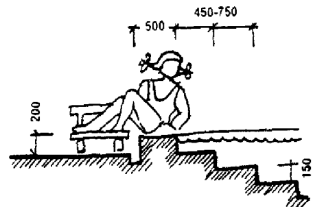
2б - с лестницей
