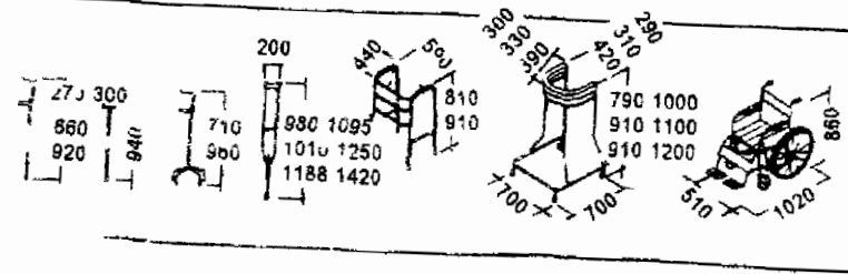
РИС 3.4 НЕОБХОДИМЫЕ ГАБАРИТЫ КОММУНИКАЦИИ УСТРОЙСТВ И СРЕДСТВ ПЕРЕДВИЖЕНИЯ ИНВАЛИДОВ
