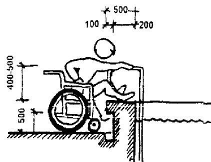
3а - без пандуса
