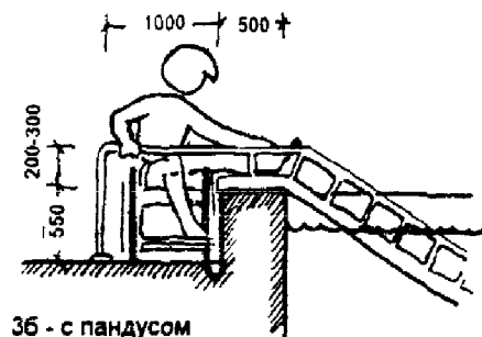
3б - с пандусом
