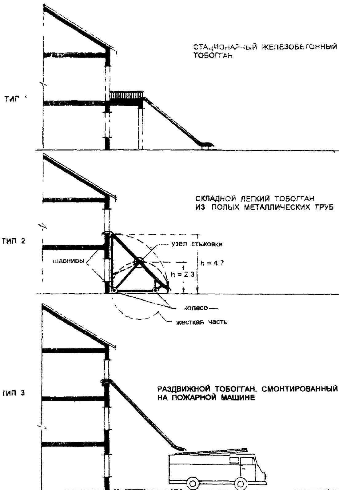
РИС 3 11 СХЕМЫ ТОБОГАНОВ
