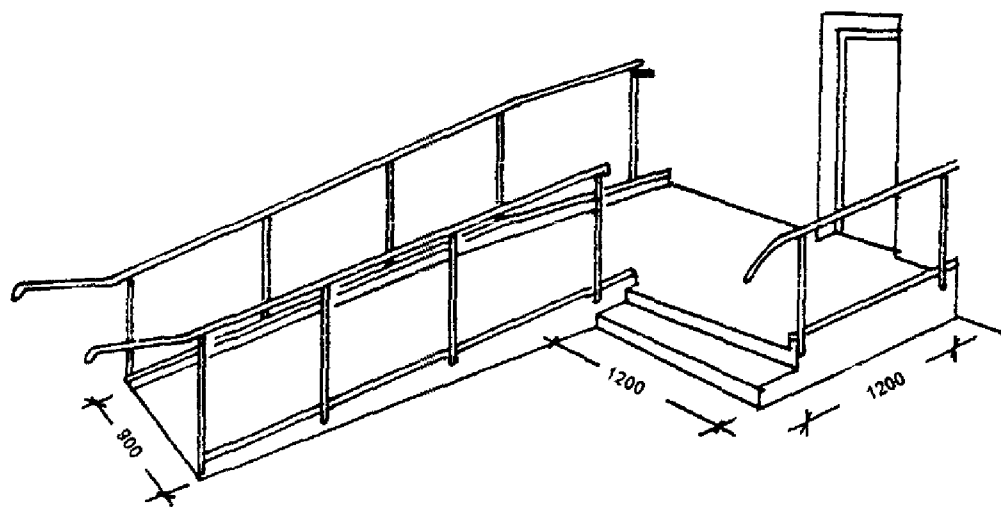
РИС.39 ПРИМЕРЫ УСТРОЙСТВА ВХОДНЫХ ЛЕСТНИЦ И ПАНДУСОВ, РАСЧИТАННЫХ НА ИНВАЛИДОВ
