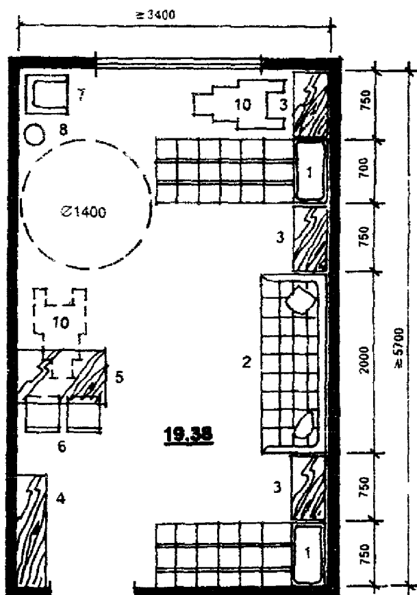
РИС 4 8 ПЛАНИРОВОЧНЫЕ СХЕМЫ СПАЛЬНЫХ КОМНАТ НА 3 И 4 МЕСТА
