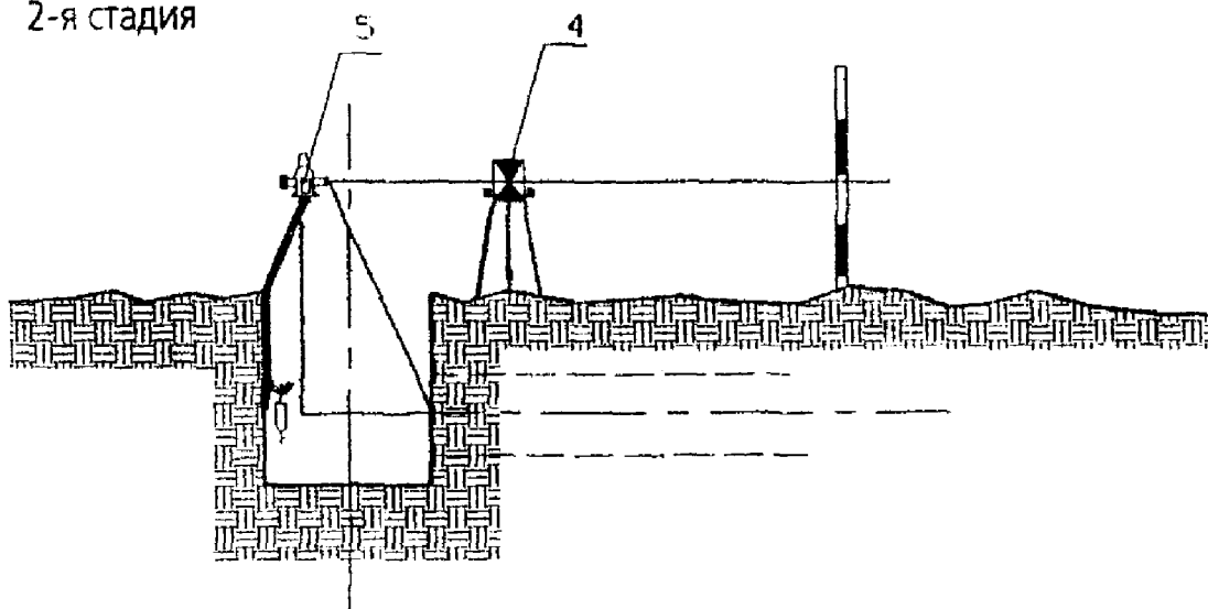
Рис. Е-1. Схема маркшейдерской привязки:
