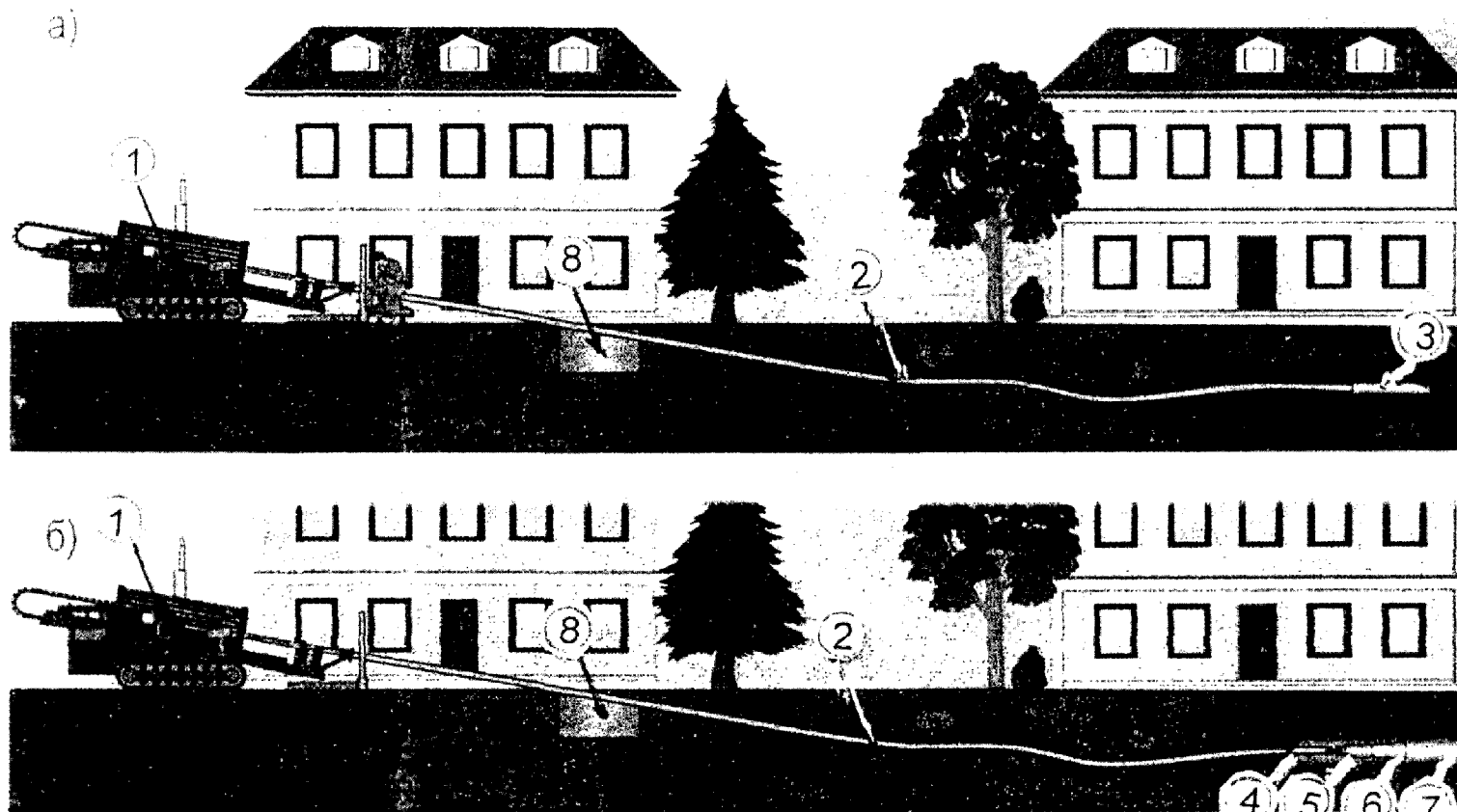
Рис.2. Конструктивно-технологическая схема установки направленного мелкого бурения
