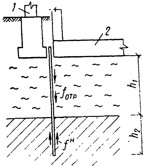
Рис 1. Разъединительная шпунтовая стенка
