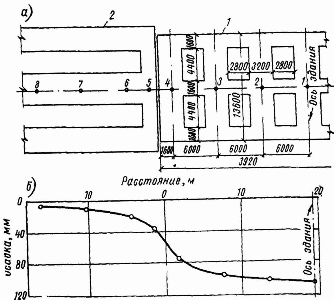
Рис 4 Схема к примеру расчета осадки
