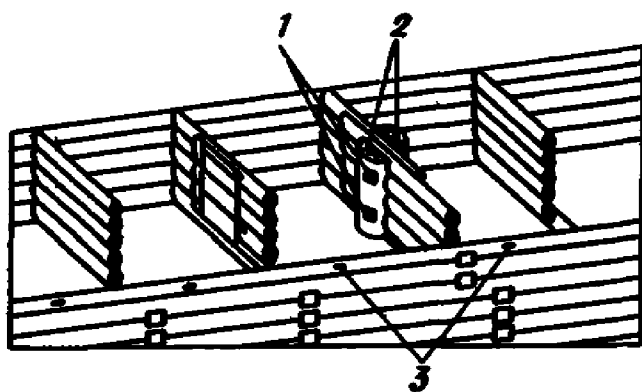
Рис. 18. Первый способ нарубки лицевых стен камеры шлюза
