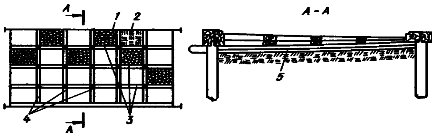
Рис. 24. Схема-ростверка
