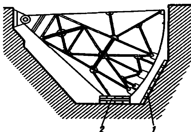
Рис 5. Схема рабочей зоны 1 — лестница; 2 — опорные клетки
