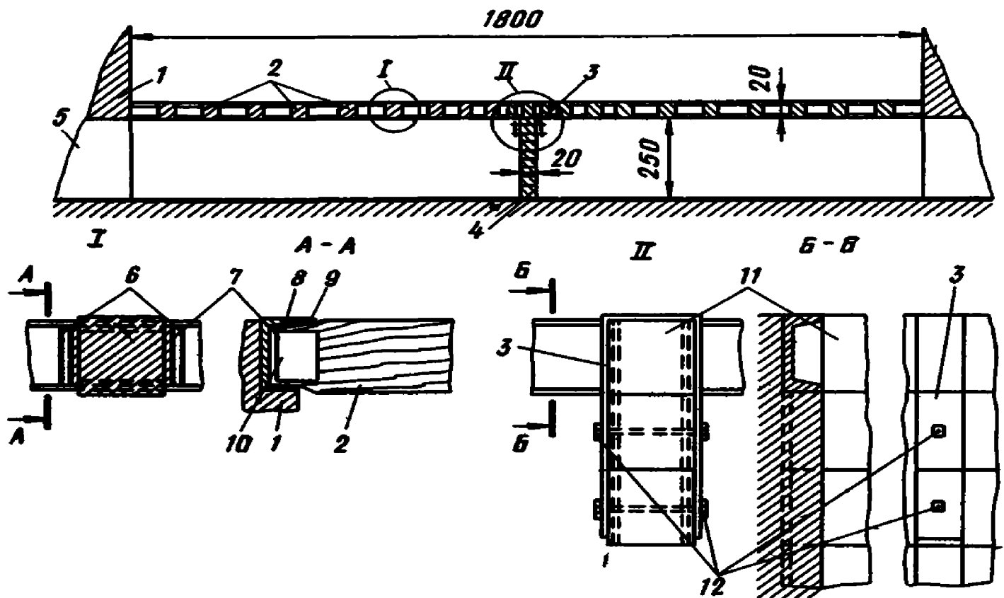
Рис. 10. Схема ниши гашения (разрезы)
