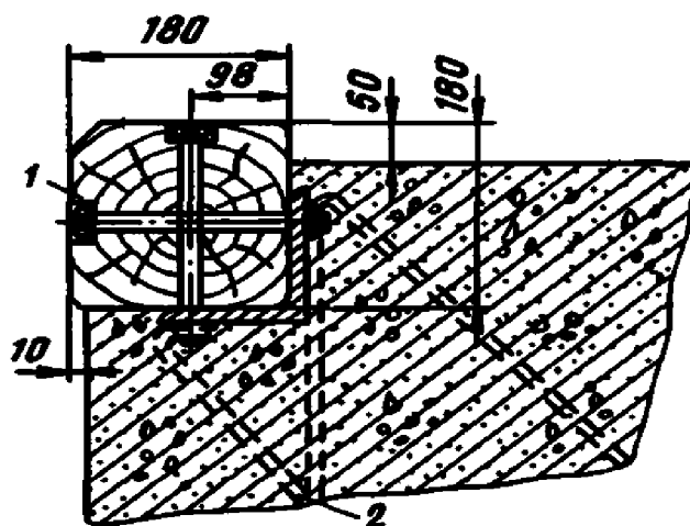
Рис. 7. Брус уплотнения порога короля 1 — брус уплотнения; 2 — анкерный болт
