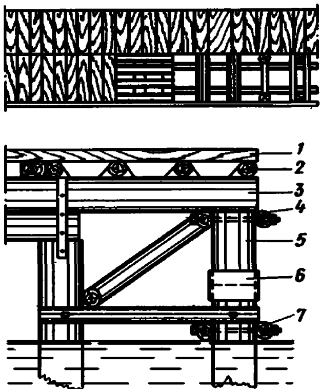
Рис 15. Схема поперечного настила
