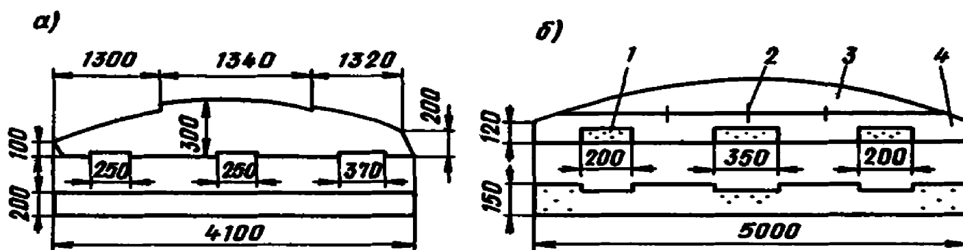
Рис. 6. Схемы шпангоутов. а — верхнего яруса; б — нижнего яруса: 1 — отверстия под заклепки, 2 — скобы для крепления брусьев, 3 — верхний брус, 4 — нижний брус
