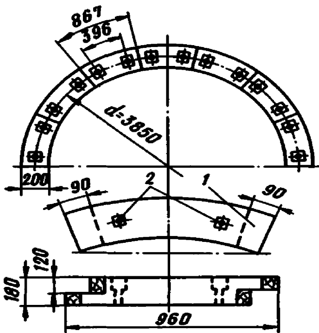
Рис. 9. Дубовое кольцо уплотнения
