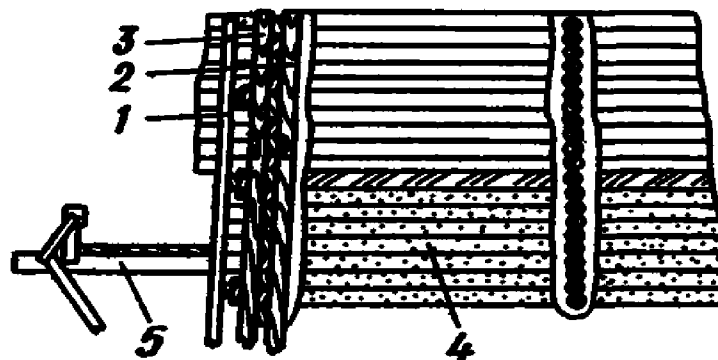
Рис. 20. Схема верхней части ряжевых стен шлюза 1 — отбойная стойка, 2 — внутренний сжим, 3 — наружный сжим, 4 — засыпка; 5 — леса на кронштейнах
