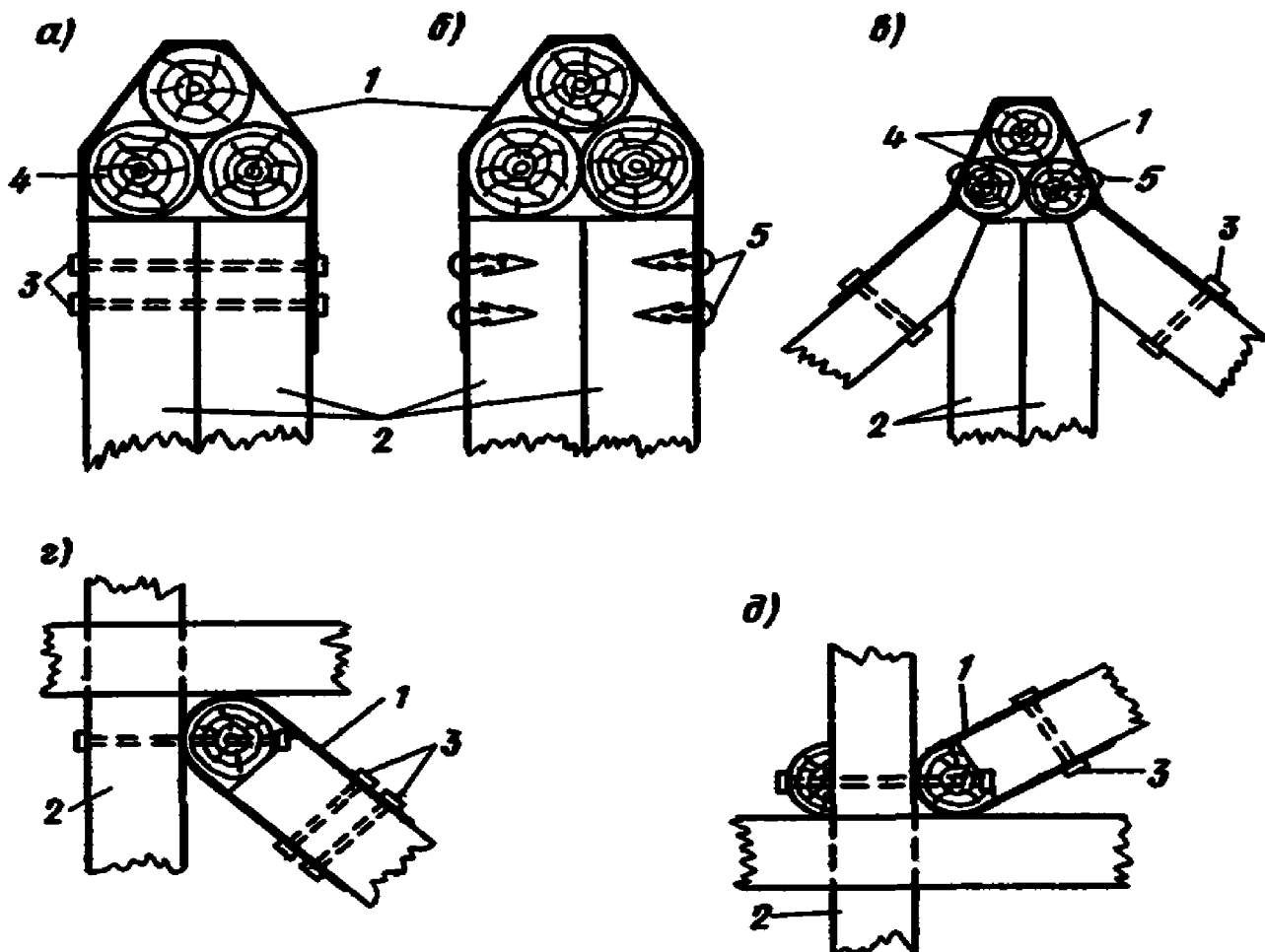
Рис. 26. Крепление хомута a — на шапочном бруске двумя болтами; б — на шапочном бруске четырьмя штырями, в — на стропилах двумя болтами и двумя штырями; г — на подкосе двумя болтами; д — на подкосе одним болтом 1 — хомуты; 2 — сваи; 3 — болты, 4 — шапочные бруска; 5 — штыри
