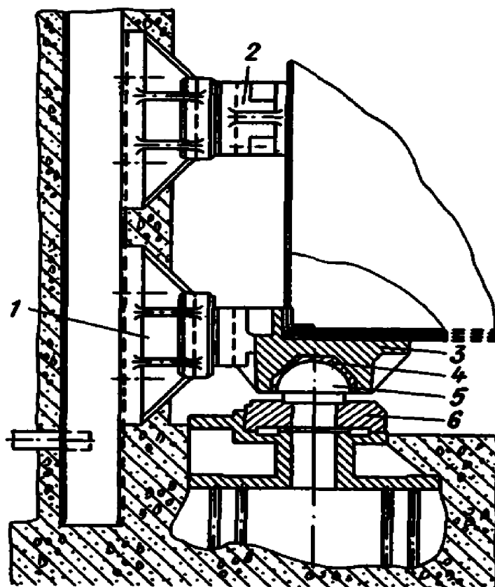
Рис. 2. Пятовое устройство ворот шлюза
