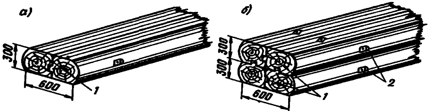
Рис. 17. Конструкции колод
