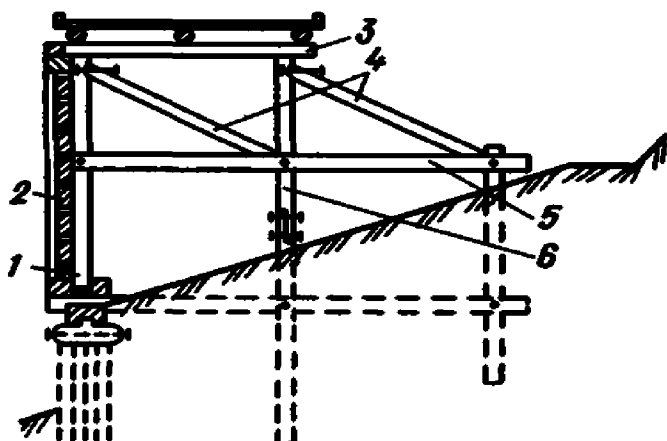
Рис. 27. Поперечный разрез эстакады
