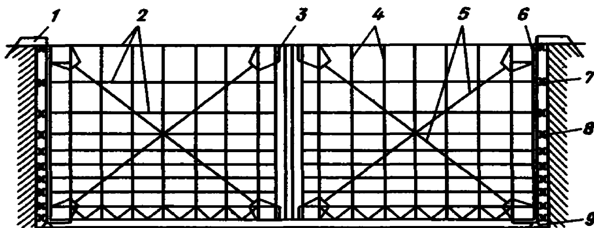
Рис 1 Схема двухстворчатых ворот шлюза
