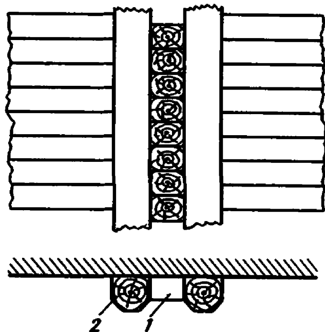
Рис. 23. Отбойная система, тип II
