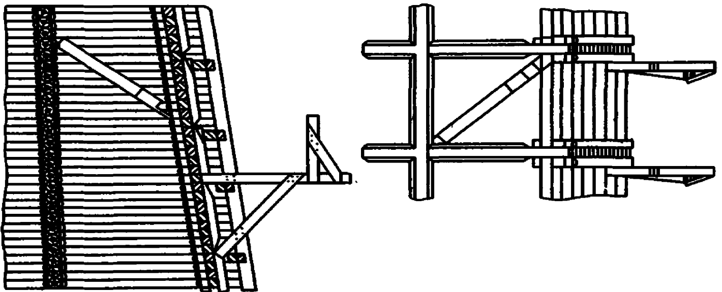
Рис. 29. Схема установки кронштейнов
