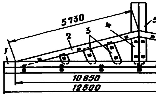
Рис 16. План королевой колоды
