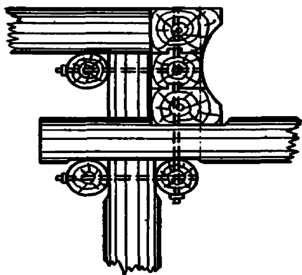
Рис. 14. Схема крепления верейльного столба
