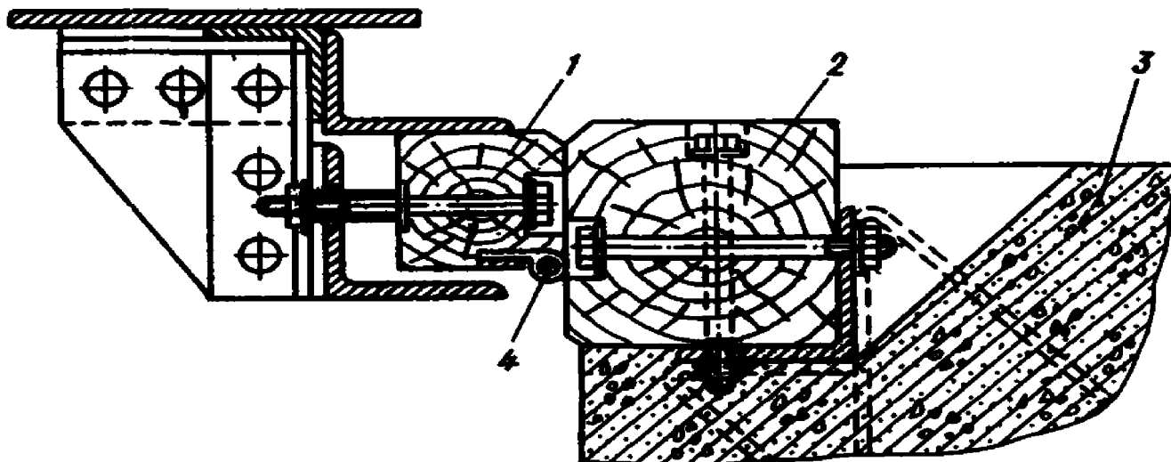
Рис. 4 Схема донного уплотнения
