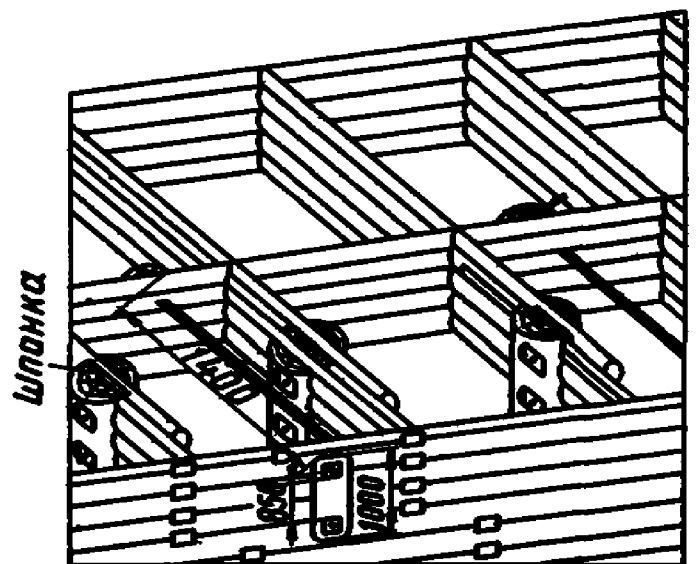
Рис. 19. Второй способ нарубки лицевых стен камеры шлюза
