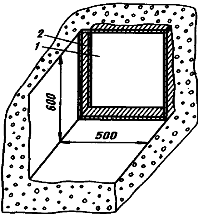
Рис. 11. Схема шпонок водопроводной галереи
