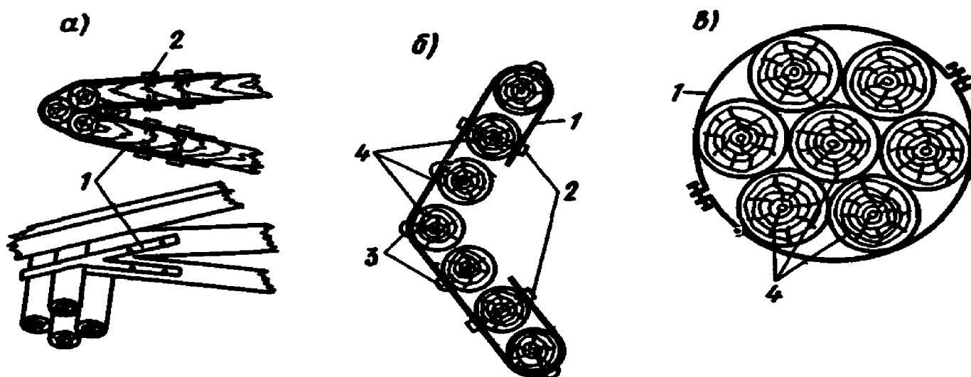
Рис. 25. Установка хомута а — на восьми болтах; б — на двух болтах и пяти штырях; в — разъемного на двух стяжных болтах 1 — хомуты; 2 — болты; 3 — штыри; 4 — сваи
