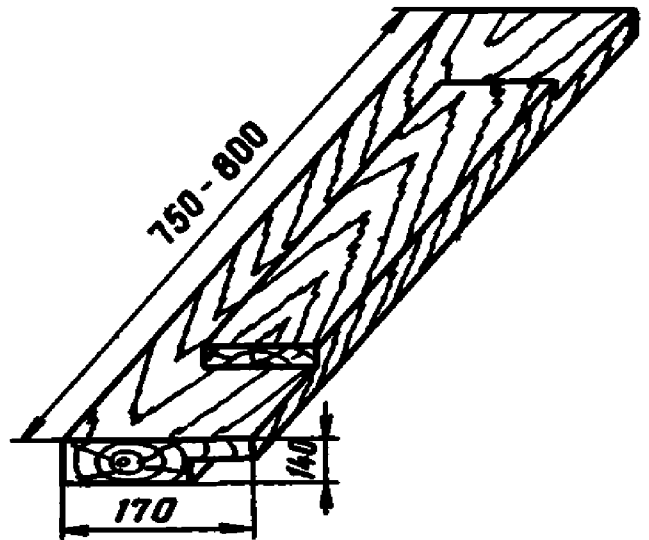
Рис. 12. Шпоночный вкладыш
