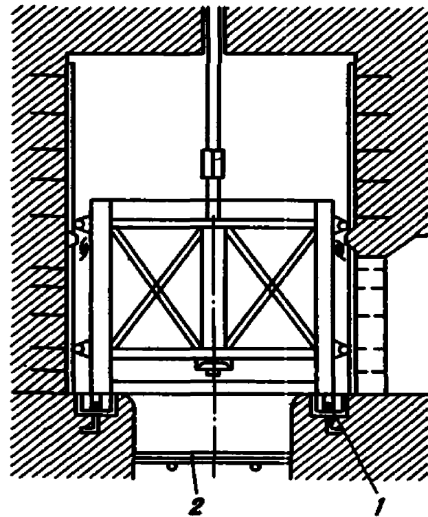
Рис. 8. Схема цилиндрического затвора
