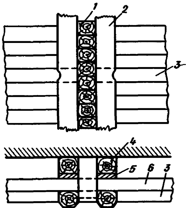
Рис. 22. Отбойная система, тип I
