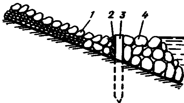
Рис. 13 Поперечный разрез забирки
