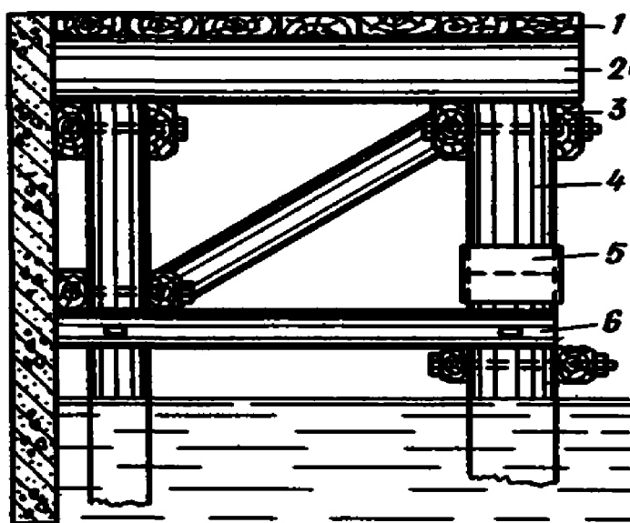
Рис. 28. Схема верхнего строения
