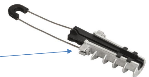
Зажим анкерный ЗАН 50-70/1500 клинового типа
